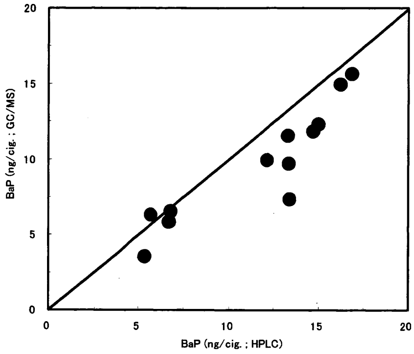
図-1c GC/MSとHPLCによるBaP測定値の関係
