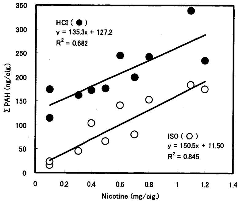
図-3 ニコチン量(表示値)と総PAH濃度の関係
