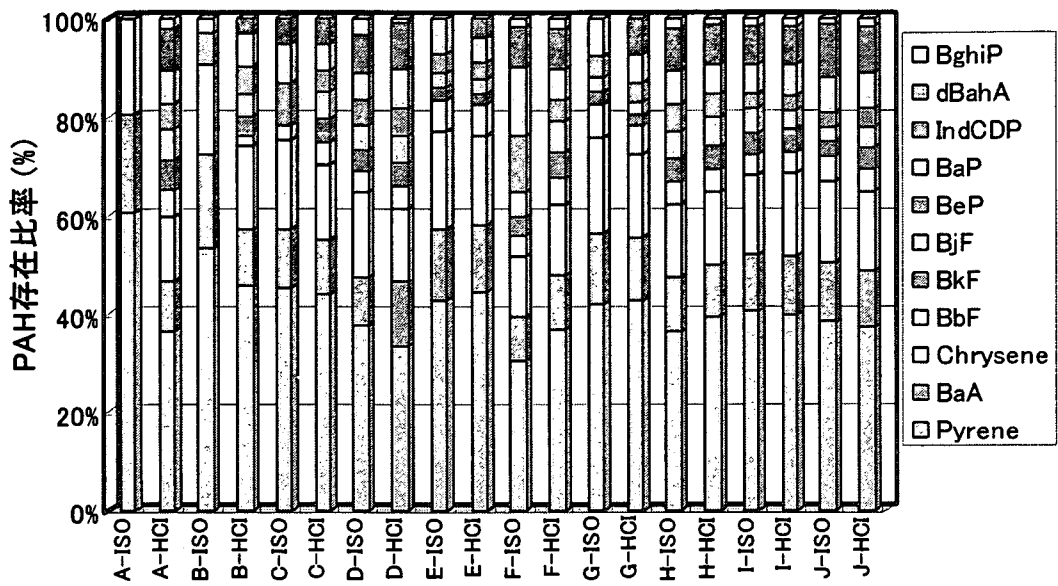
図-2 たばこ主流煙中の各PAH存在比率
