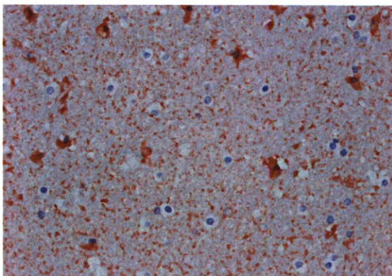
図 3 A：脳症による突然死症例の脳幹部。GFAP 染色で、アストロサイトは断裂 (clasmatodendrosis) が著しい。B：対照。
