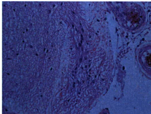
図 2 LGH は脳形成異常で脳軟膜内に突出した神経組織で、アストロサイト、時には神経細胞の迷入を認める。これは、脳底部、特に視床下部の下面によく認められる。
