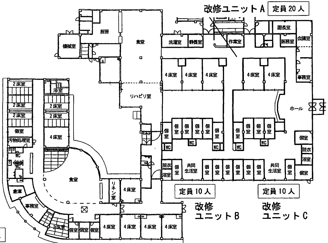
図表 1-82 本体施設の平面図 1/600
