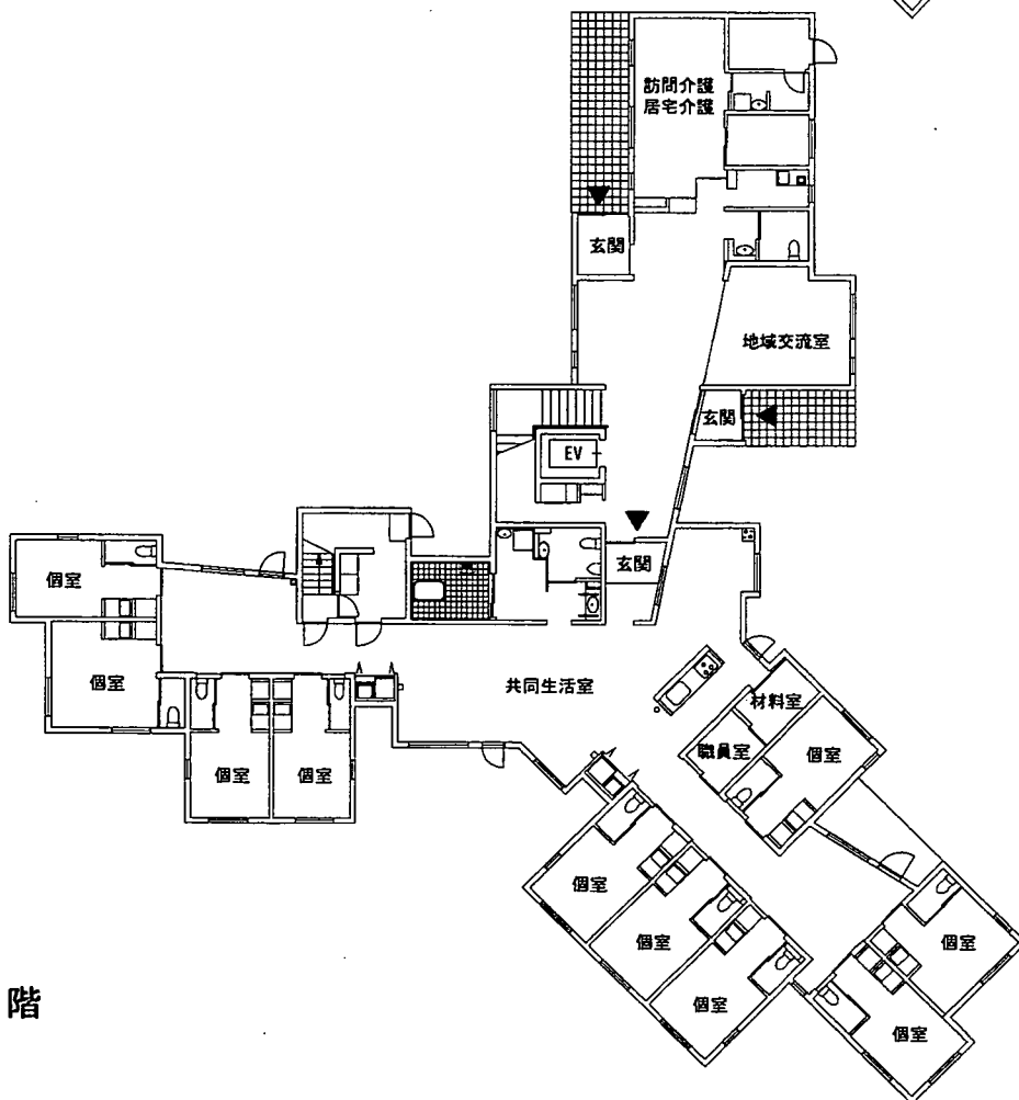
図表1-6 サテライトの平面図 1/300
