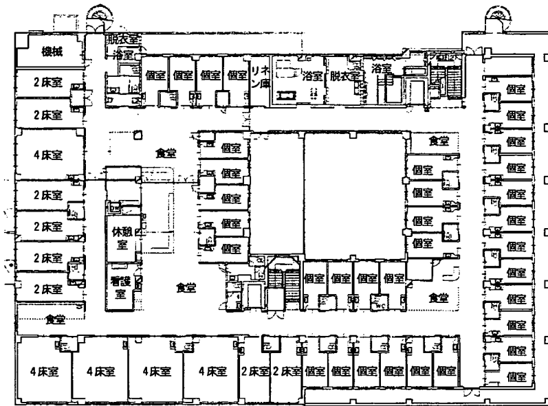
2階平面図
