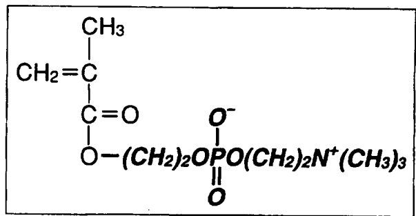
図5 MPCの構造
