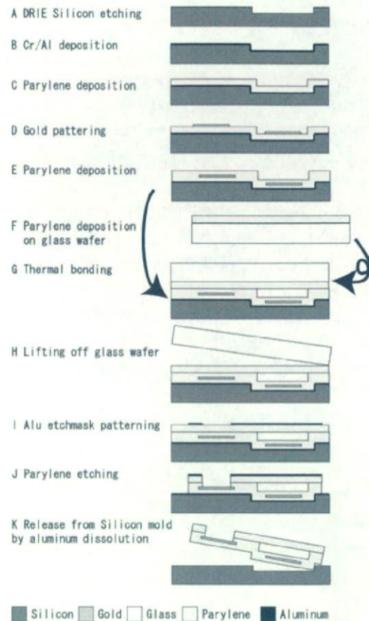
図17 貼り合わせ法の詳細プロセス。溝型構造を作成するために、まずDeepRIEによってシリコンウェハに溝を掘る。
