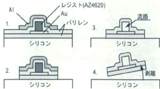
図4: 微小流路を備えた柔軟神経電極の作成方法。厚膜レジストを犠牲層としてシリコンウェハ上で作成する。最終的にはレジストをアセトンで除去し、ウェハから剥離して完成する。
