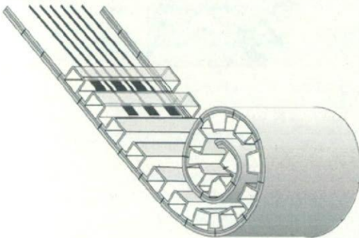
図12: 今回提案する再生型電極。フィルム上に多数の流路構造を並べ、巻いて固定してから流路内の厚膜レジストを除去する。各流路内には複数の電極を配置可能である。
