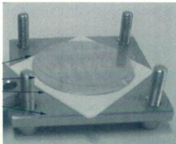
図16 貼り合わせ法において使用する器具。2枚のステンレス板で2枚のパリレンを強力に挟みこみ、そのまま約150℃の炉で熱する。
