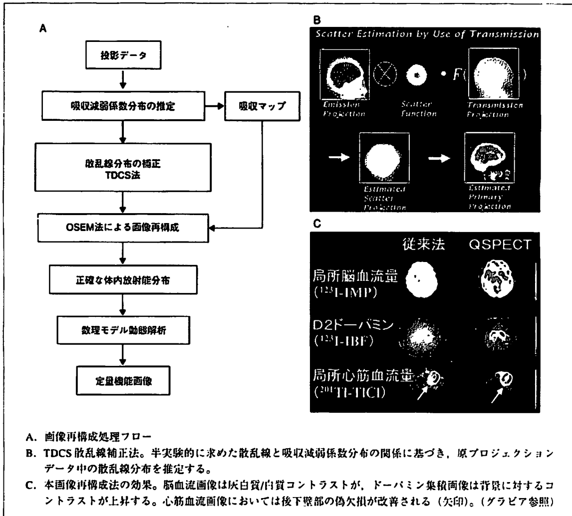
図⑥ 定量的SPECT画像再構成
