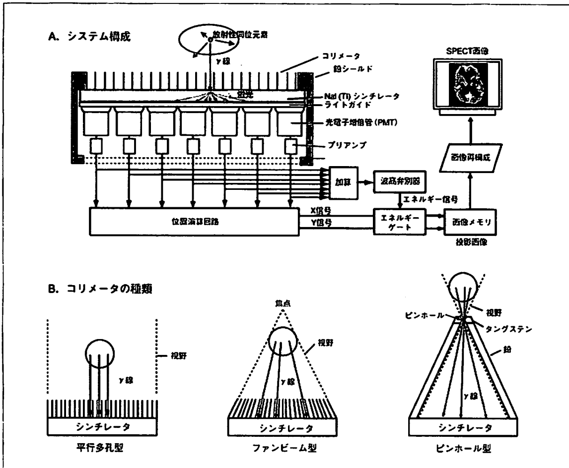
図2 SPECT装置
