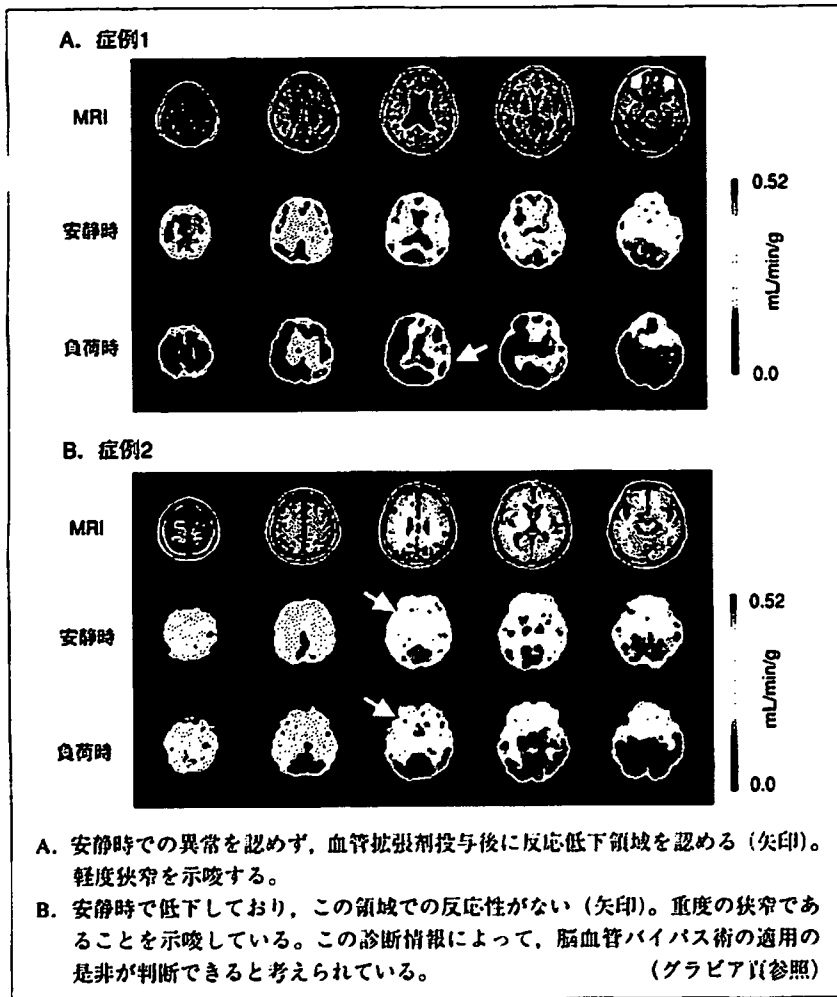
図① ^{125}\text{I} -IMPを使って得た安静時と血管拡張剤投与後の脳血流画像の例
