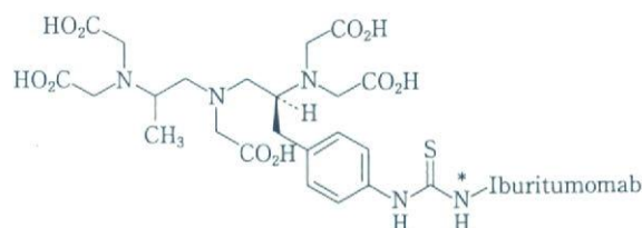
図3 Ibiritumomab Tiuxetan(イブリツモマブ チウキセタン)の構造(日本承認申請中)
