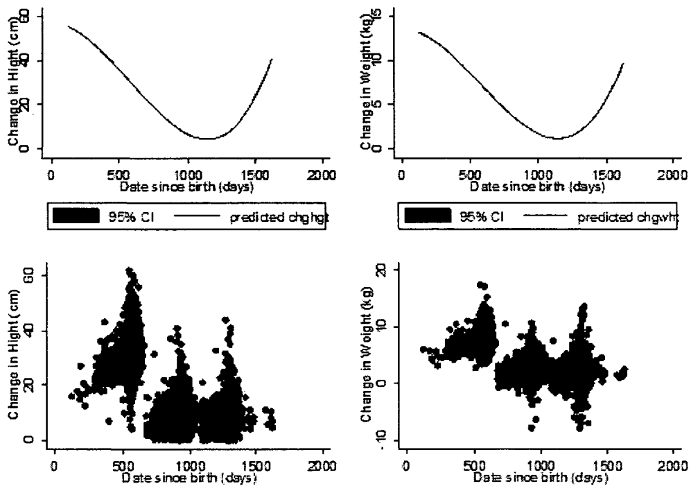
図8 身長と体重の変化のプロット図と統計的推定図（外れ値除くサンプル）
