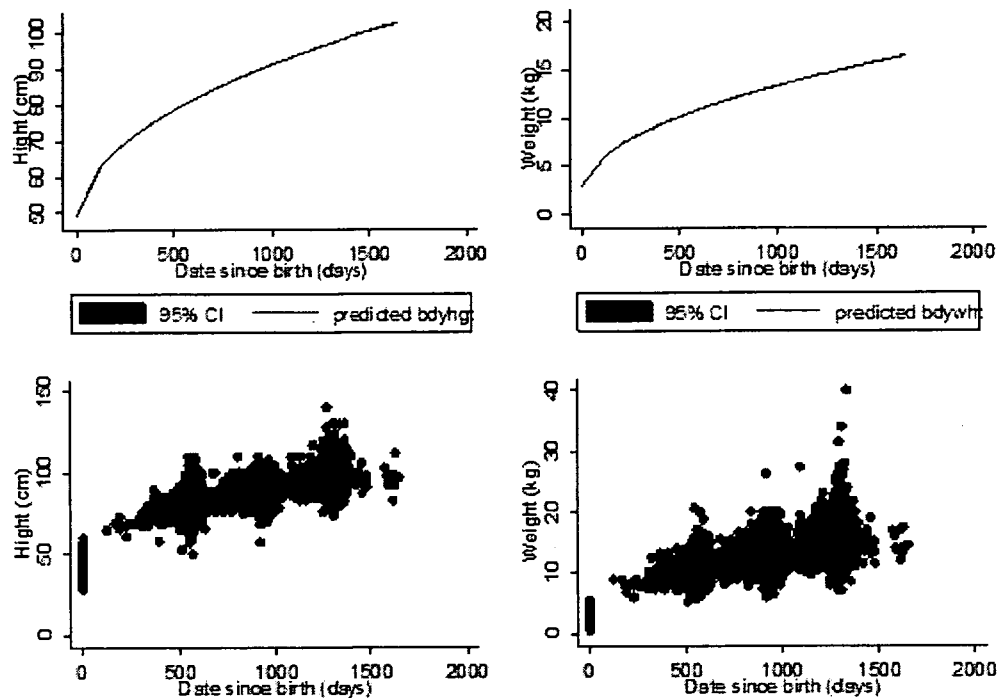
図4 身長と体重のプロット図と統計的推定図 (外れ値除くサンプル)
