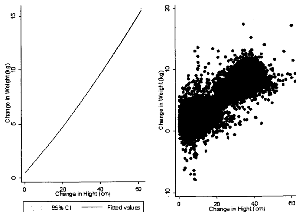
図10 身長と体重の変化のクロスプロット図 (外れ値除くサンプル)
