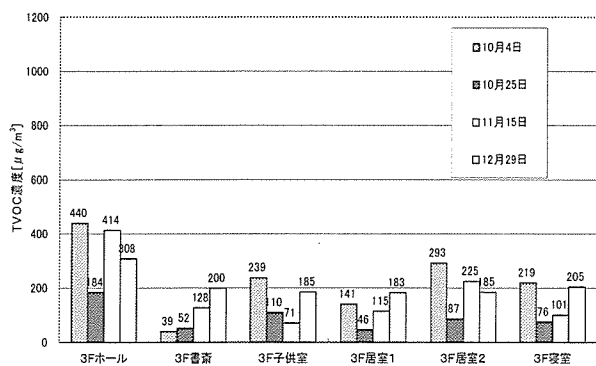
図-5 各居室のVOC濃度(3F)
