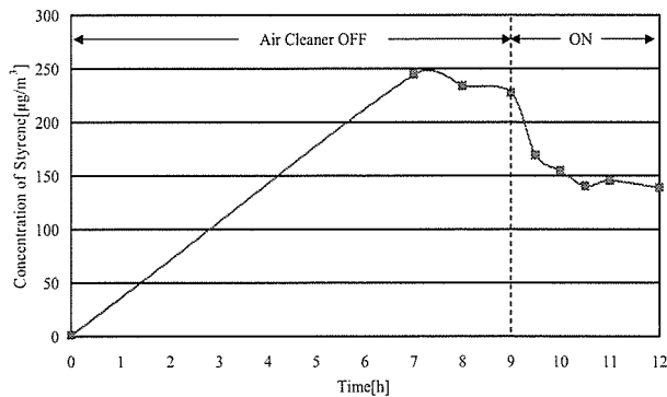
図一 2 3 機器運転に伴うStyrene濃度の経時変化 (5th)
