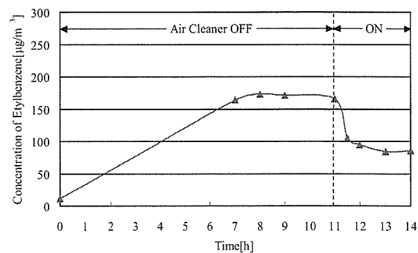
図一 2 4 機器運転に伴うEthylbenzene濃度の経時変化 (6th)
