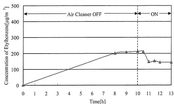
図一 1 8 機器運転に伴うEthylbenzene濃度の経時変化 (4th)
