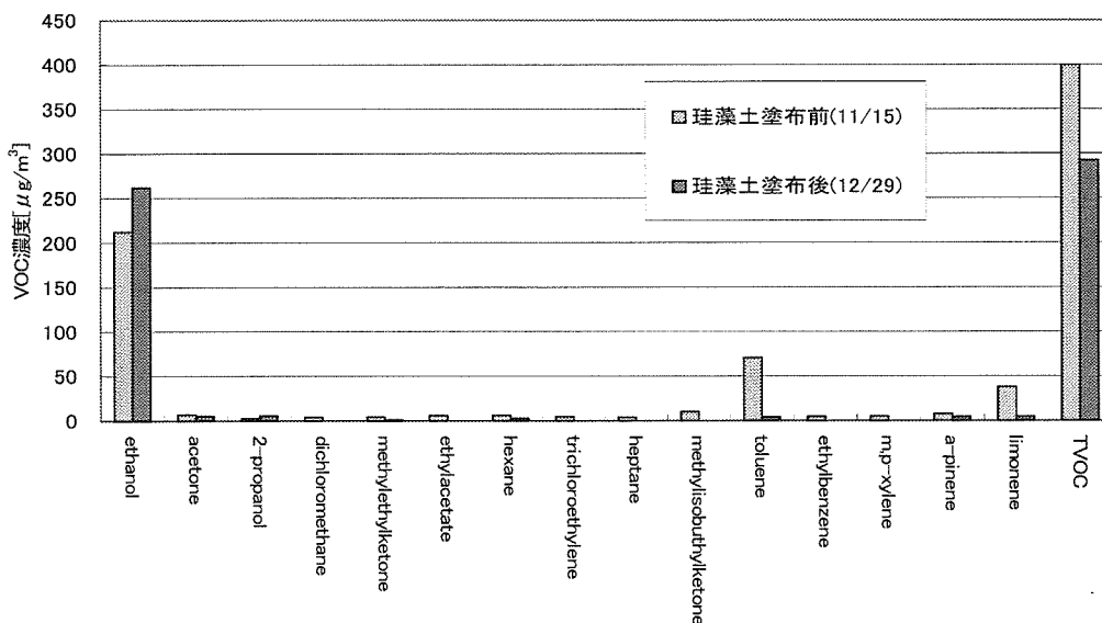
図-10 珪藻土塗布前後の VOC 濃度 (2F 玄関ホール)
