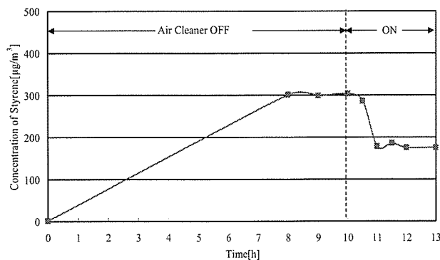
図一 2 0 機器運転に伴うStyrene濃度の経時変化 (4th)
