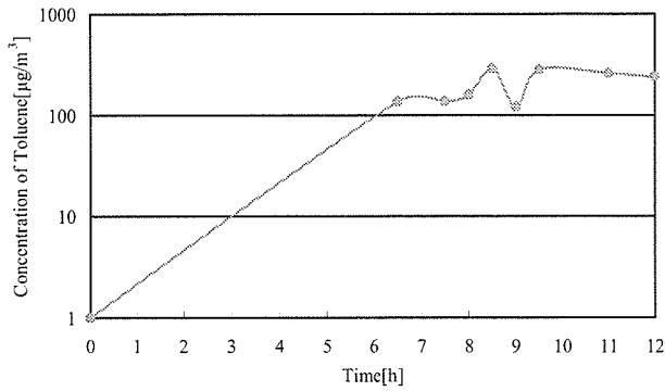
図-11 Toluene 定常状態確認試験
