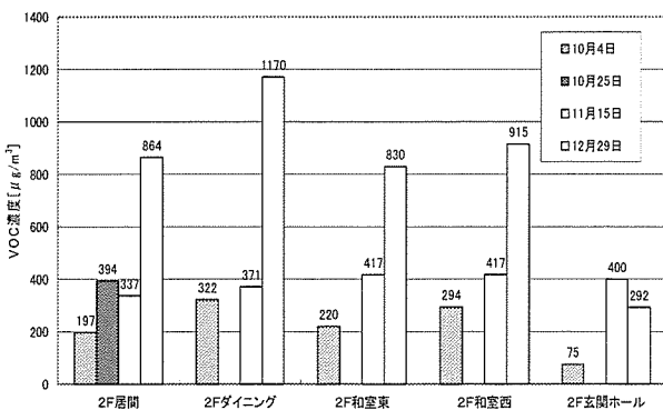
図-8 各居室のホルムアルデヒド濃度(2F)
