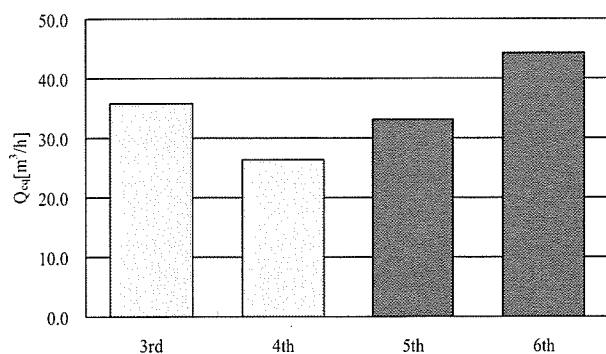
図-30 Styrene 相当換気量
