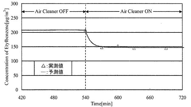
図-40 Ethylbenzene濃度実測値と濃度予測値との比較 (4th)
