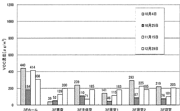
図-7 各居室のホルムアルデヒド濃度(3F)
