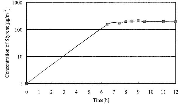
図-14 Styrene 定常状態確認試験
