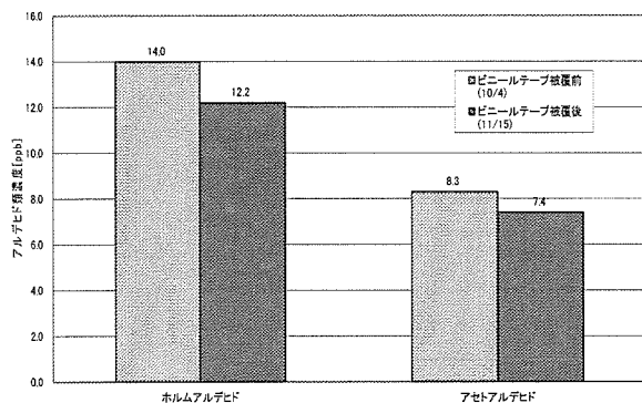
図-14 ビニールテープ被覆前後のアルデヒド濃度
