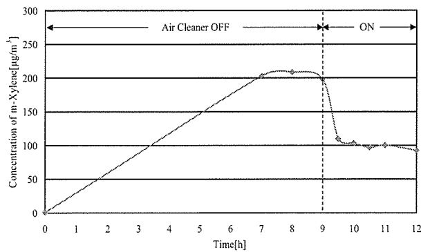
図一 2 2 機器運転に伴うm-Xylene濃度の経時変化 (5th)
