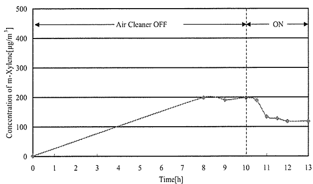
図一 1 9 機器運転に伴うm-Xylene濃度の経時変化 (4th)
