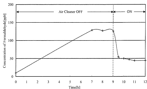
図-9 機器運転に伴う Formaldehyde 濃度の経時変化 (5th)
