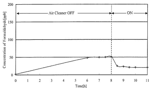
図-5 機器運転に伴う Formaldehyde 濃度の経時変化 (1st)
