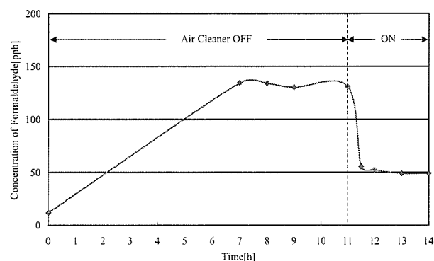
図-10 機器運転に伴う Formaldehyde 濃度の経時変化 (6th)
