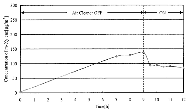
図一 1 7 機器運転に伴うStyrene濃度の経時変化 (3rd)
