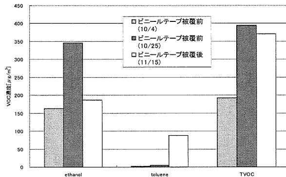
図-15 ビニールテープ被覆前後の VOC 濃度
