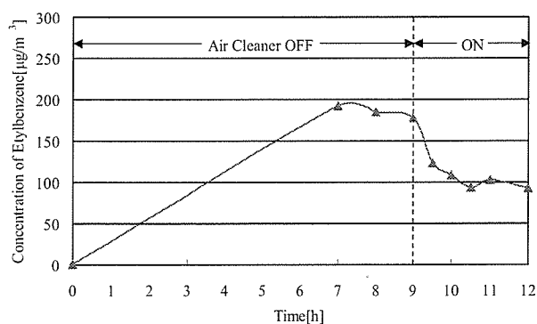
図一 2 1 機器運転に伴うEthylbenzene濃度の経時変化 (5th)
