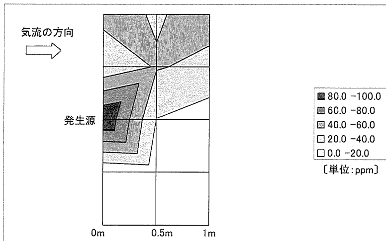
図 27 実験 3 の床上 0.7m における乱流モデルで得られた気中酢酸エチル濃度の分布
