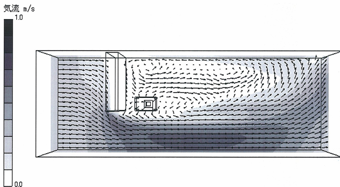
図 14 実験 1 の床上 0.9mにおける気流の方向と速度分布の層流モデル解析結果
