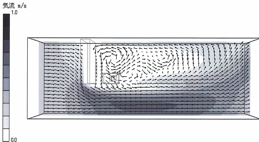
図 13 実験 1 の床上 0.9mにおける気流の方向と速度分布の乱流モデル解析結果
