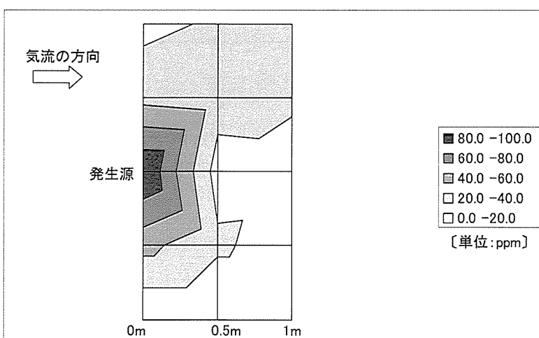
図 19 実験 2 の床上 0.7m における層流モデルで得られた気中酢酸エチル濃度の分布
