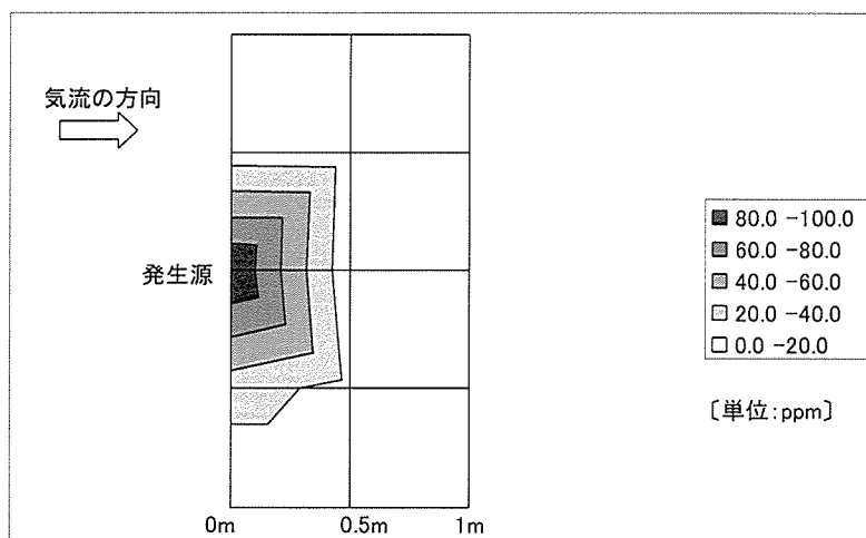
図 6 実験 1 の床上 0.7m における層流モデルで得られた気中酢酸エチル濃度の分布
