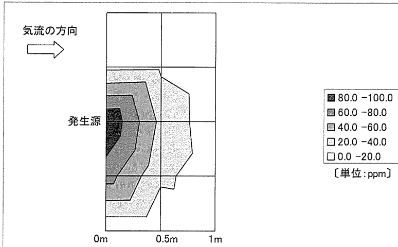
図 20 実験 2 の床上 0.9m における実測値の気中酢酸エチル濃度の分布
