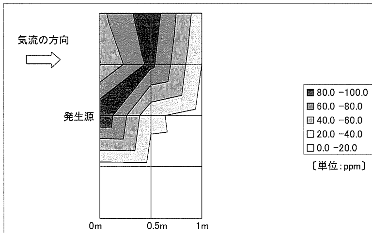
図 8 実験 1 の床上 0.9m における乱流モデルで得られた気中酢酸エチル濃度の分布
