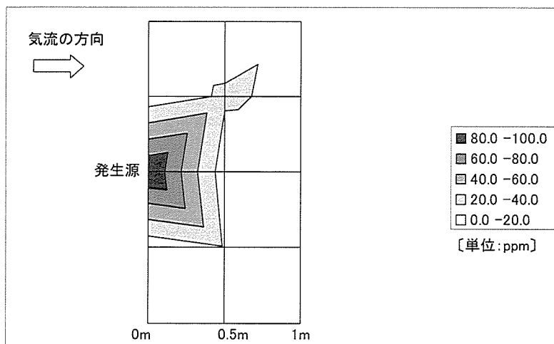
図 28 実験 3 の床上 0.7m における層流モデルで得られた気中酢酸エチル濃度の分布
