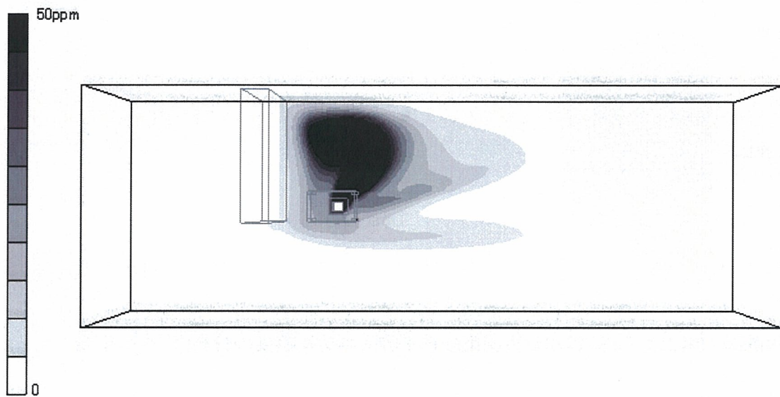
図 15 実験 1 の床上 0.9mにおける酢酸エチルの濃度分布の乱流モデル解析結果
