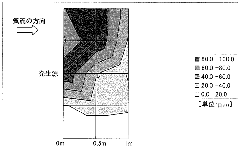
図 21 実験 2 の床上 0.9m における乱流モデルで得られた気中酢酸エチル濃度の分布
