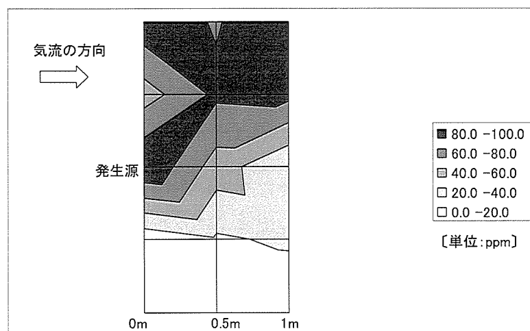
図 30 実験 4 の床上 0.7m における乱流モデルで得られた気中酢酸エチル濃度の分布
