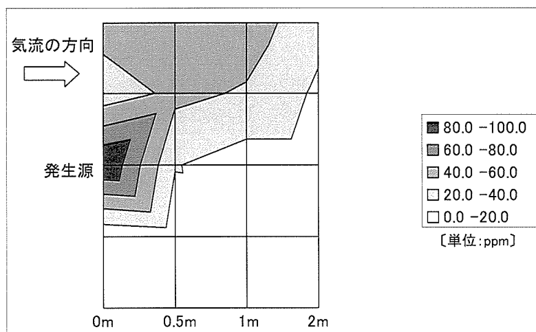
図 36 実験 6 の床上 0.7m における乱流モデルで得られた気中酢酸エチル濃度の分布
