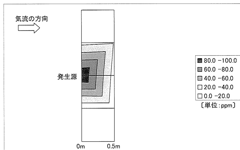
図 25 実験 2 の床上 1.1m における層流モデルで得られた気中酢酸エチル濃度の分布
