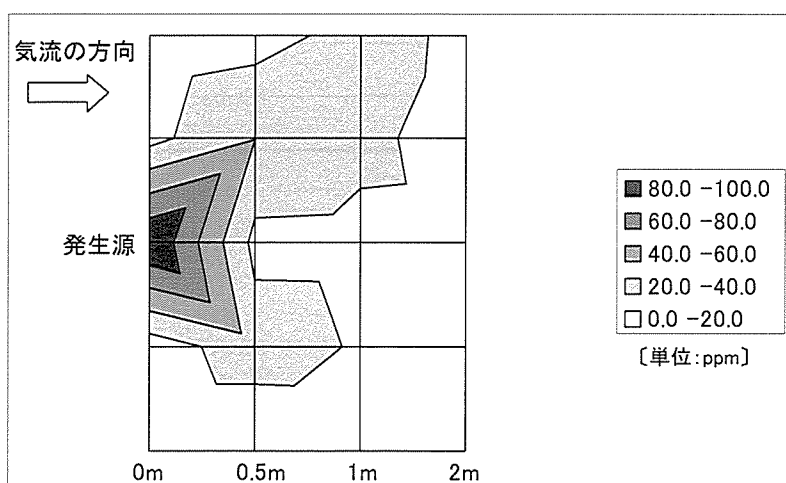
図 40 実験 7 の床上 0.7m における層流モデルで得られた気中酢酸エチル濃度の分布
