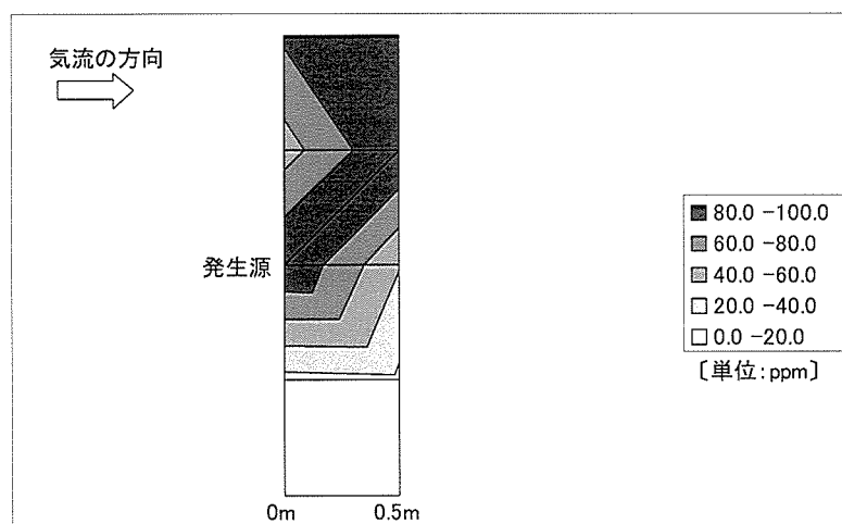
図 24 実験 2 の床上 1.1m における乱流モデルで得られた気中酢酸エチル濃度の分布
