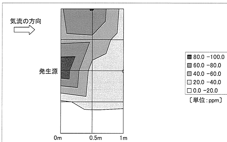
図 18 実験 2 の床上 0.7m における乱流モデルで得られた気中酢酸エチル濃度の分布
