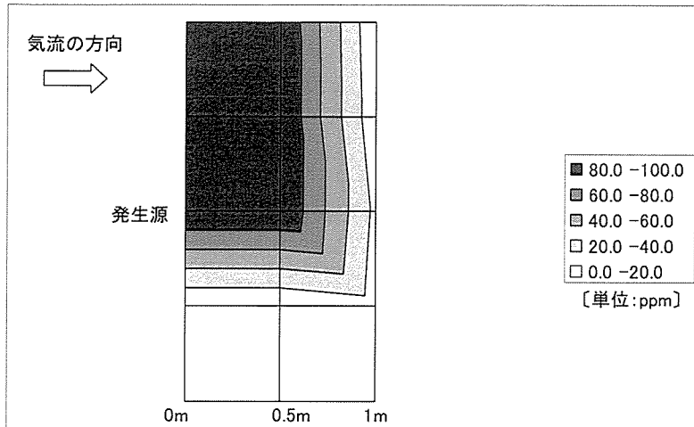
図 32 実験 5 の床上 0.7m における実測値の気中酢酸エチル濃度の分布
