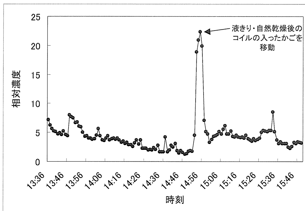
図 41 作業環境測定の実験点No.5におけるリアルタイム連続測定の結果
