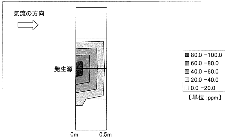
図 10 実験 1 の床上 1.1m における実測値の気中酢酸エチル濃度の分布
