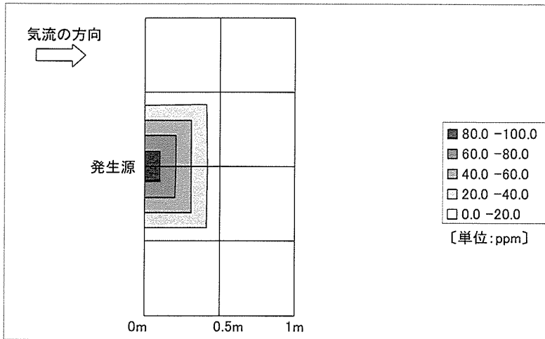
図 26 実験 3 の床上 0.7m における実測値の気中酢酸エチル濃度の分布
