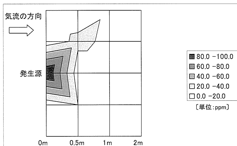
図 37 実験 6 の床上 0.7m における層流モデルで得られた気中酢酸エチル濃度の分布
