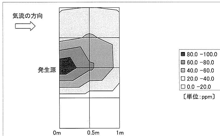
図 29 実験 4 の床上 0.7m における実測値の気中酢酸エチル濃度の分布
