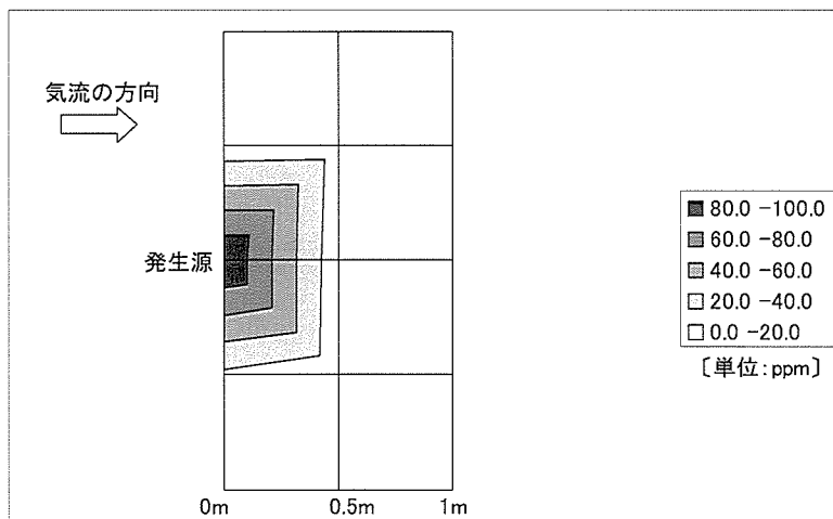
図 9 実験 1 の床上 0.9m における層流モデルで得られた気中酢酸エチル濃度の分布
