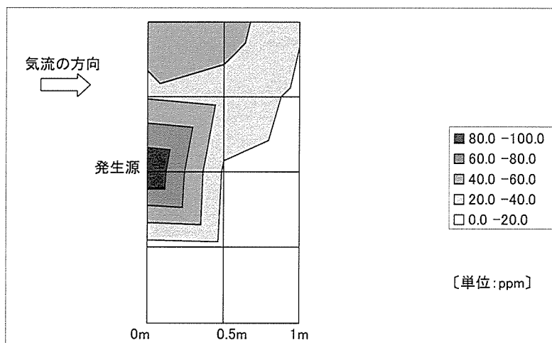
図 5 実験 1 の床上 0.7m における乱流モデルで得られた気中酢酸エチル濃度の分布
