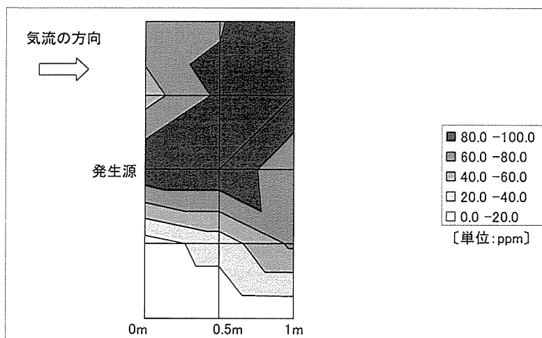
図 33 実験 5 の床上 0.7m における乱流モデルで得られた気中酢酸エチル濃度の分布
