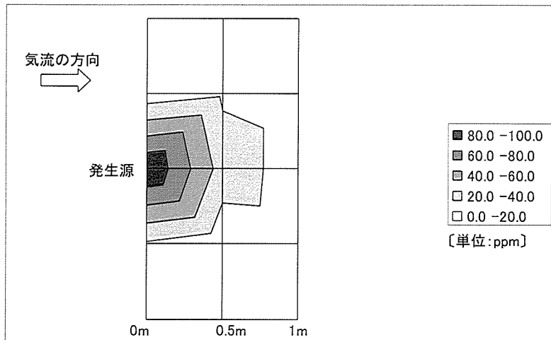
図 4 実験 1 の床上 0.7m における実測値の気中酢酸エチル濃度の分布
