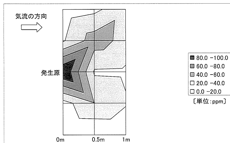
図 31 実験 4 の床上 0.7m における層流モデルで得られた気中酢酸エチル濃度の分布
