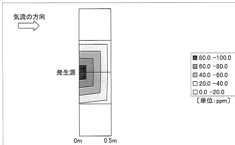
図 23 実験 2 の床上 1.1m における実測値の気中酢酸エチル濃度の分布
