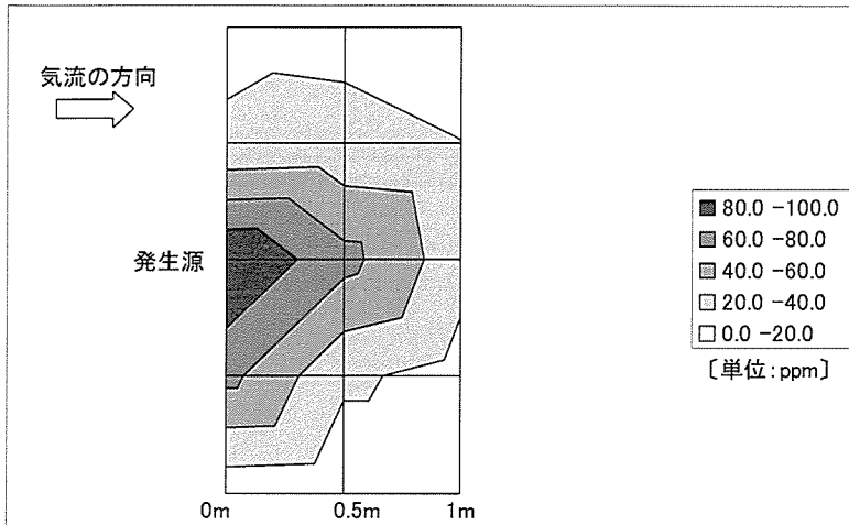
図 17 実験 2 の床上 0.7m における実測値の気中酢酸エチル濃度の分布
