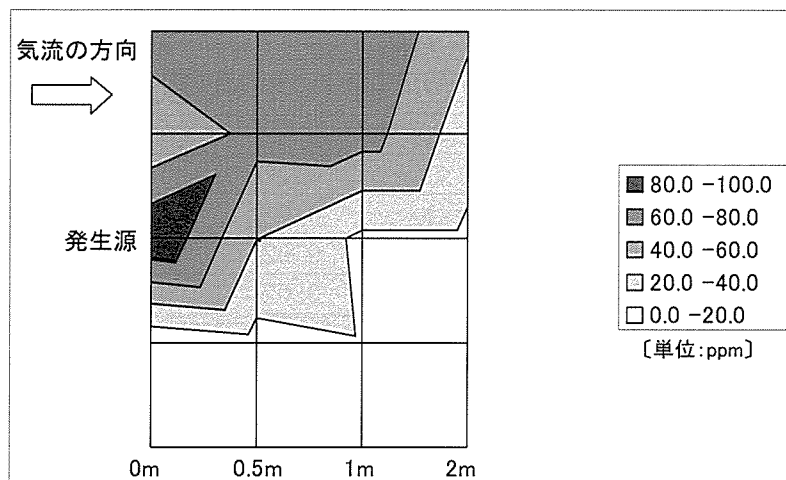
図 39 実験 7 の床上 0.7m における乱流モデルで得られた気中酢酸エチル濃度の分布
