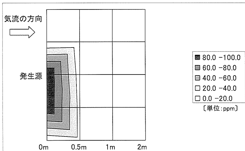
図 35 実験 6 の床上 0.7m における実測値の気中酢酸エチル濃度の分布
