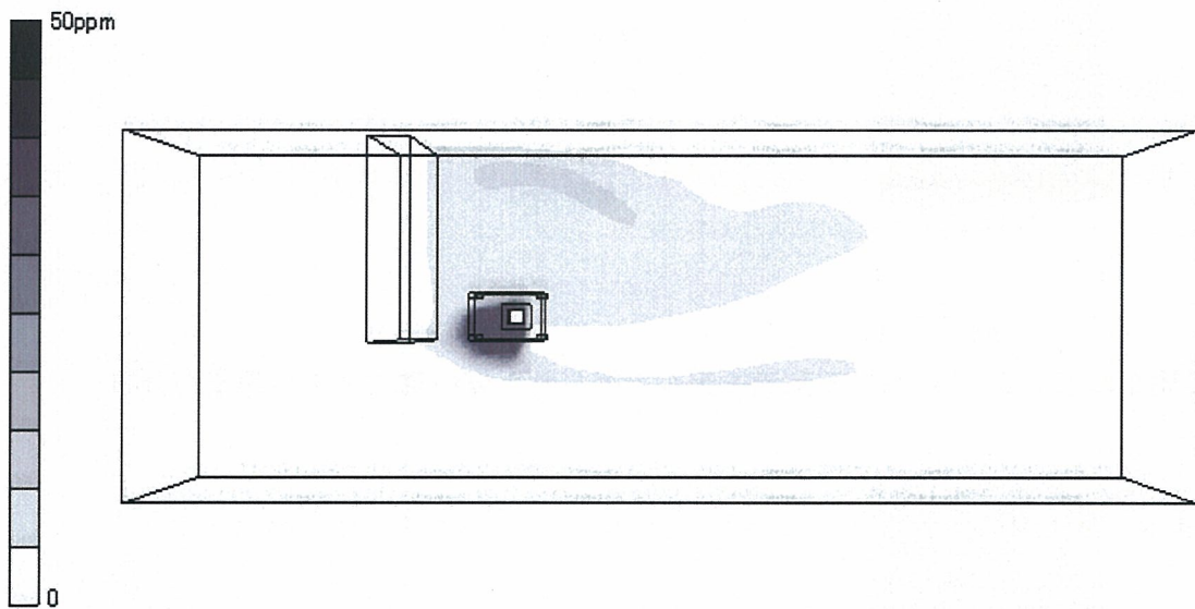
図 16 実験 1 の床上 0.9mにおける酢酸エチルの濃度分布の層流モデル解析結果
