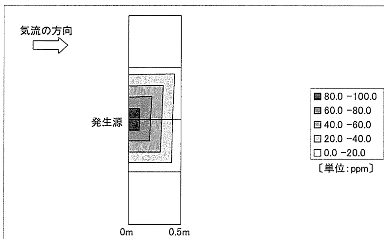
図 12 実験 1 の床上 1.1m における層流モデルで得られた気中酢酸エチル濃度の分布
