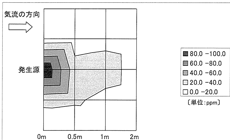
図 38 実験 7 の床上 0.7m における実測値の気中酢酸エチル濃度の分布
