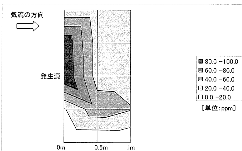
図 34 実験 5 の床上 0.7m における層流モデルで得られた気中酢酸エチル濃度の分布
