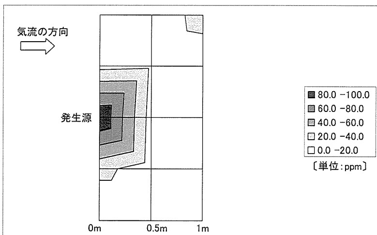
図 22 実験 2 の床上 0.9m における層流モデルで得られた気中酢酸エチル濃度の分布
