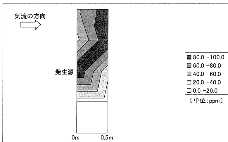
図 11 実験 1 の床上 1.1m における乱流モデルで得られた気中酢酸エチル濃度の分布
