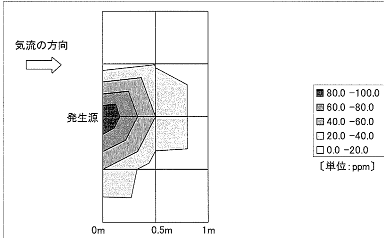
図 7 実験 1 の床上 0.9m における実測値の気中酢酸エチル濃度の分布
