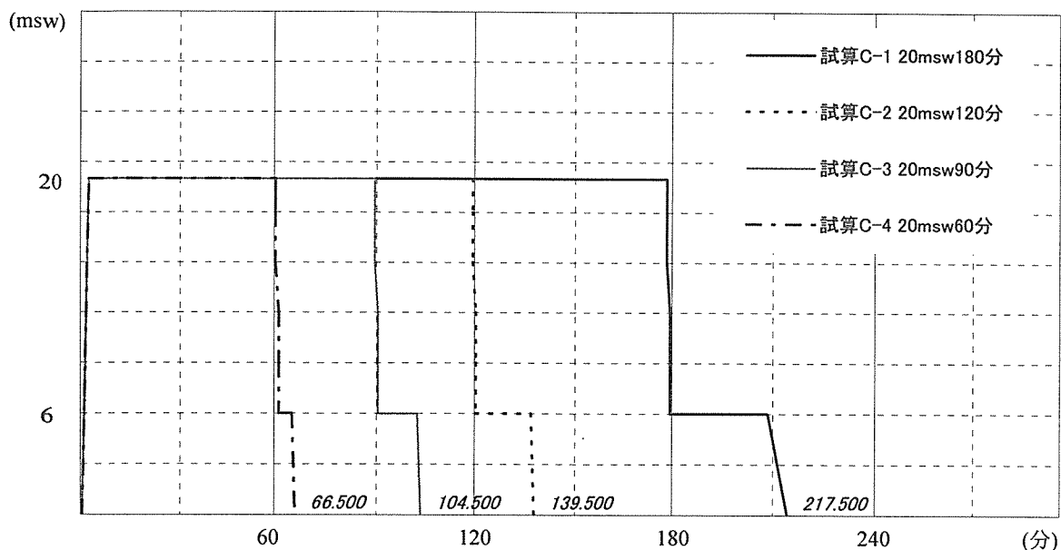
図3-15 空気減圧過程図 (20msw)-まとめ
