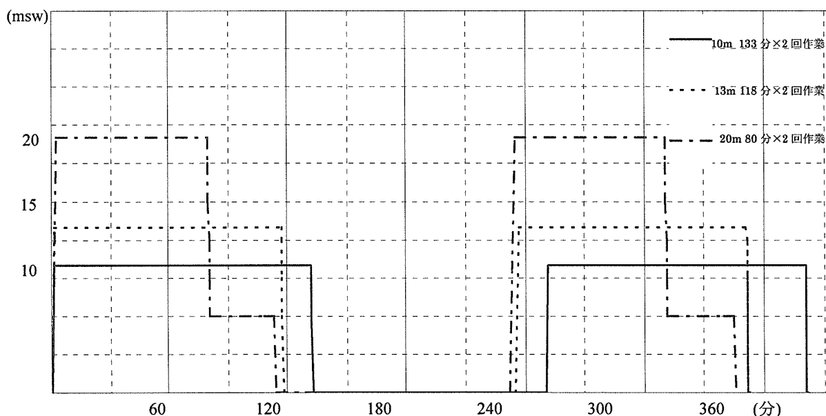
図3-22 空気減圧過程図(40msw,90分)
