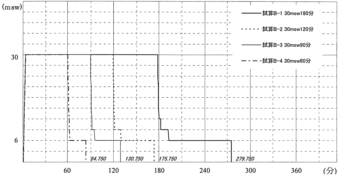
図3-10空気減圧過程図(30msw)-まとめ
