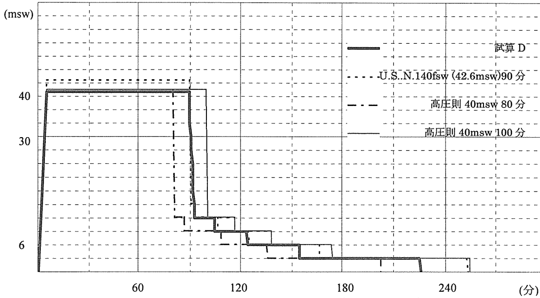
図3-20 空気減圧過程図(40msw,90分)
