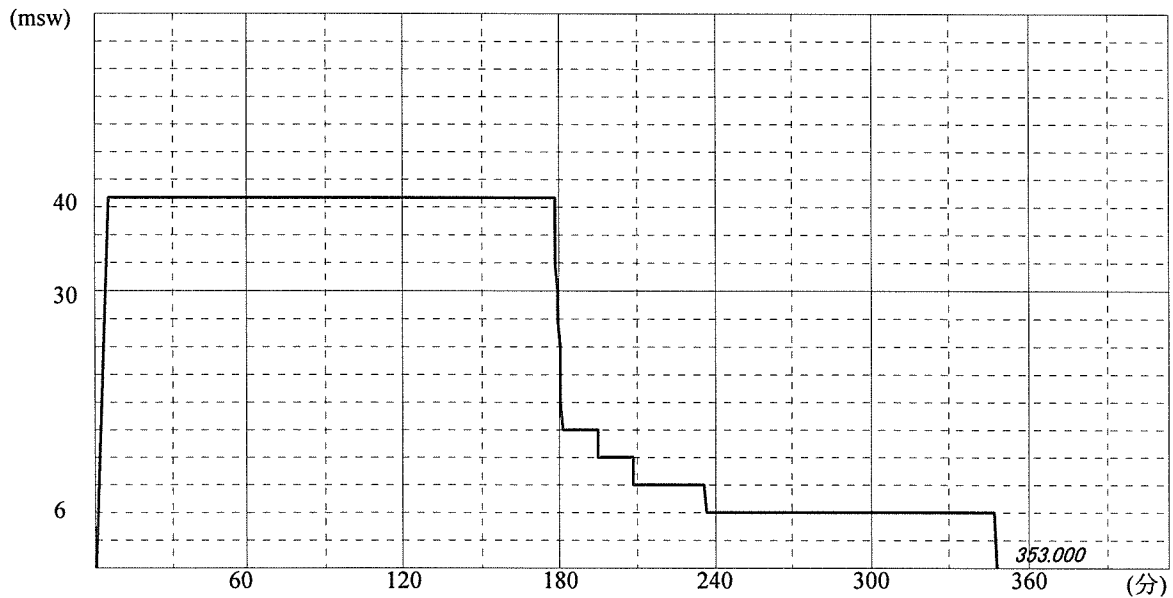
図 3-2 空気減圧過程図 (40msw,180 分)
