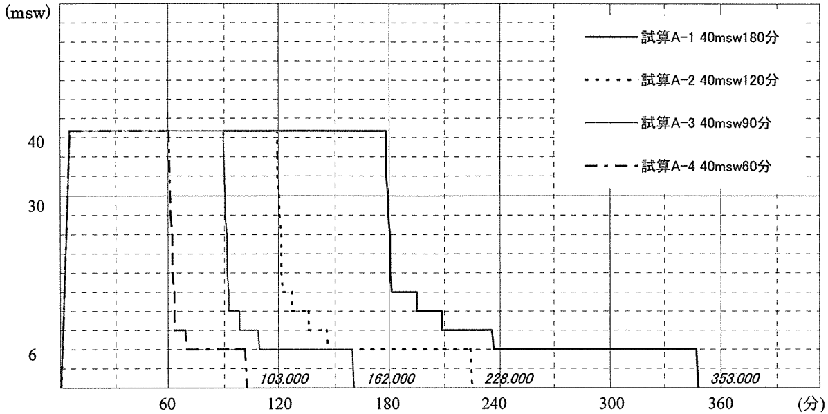
図3-4 空気減圧過程図 (40msw)-まとめ
