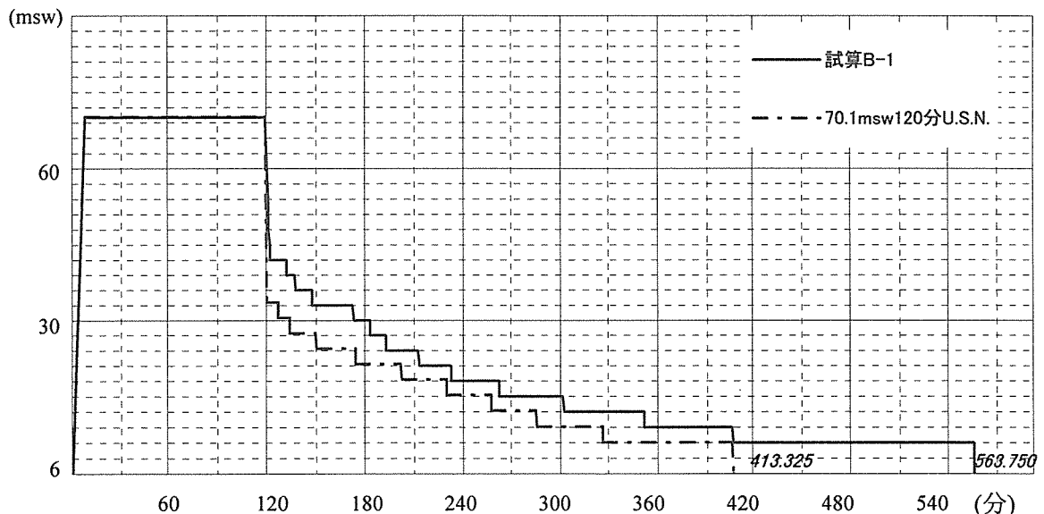
図2-35 ヘリオックス減圧過程図(70msw,120分)
