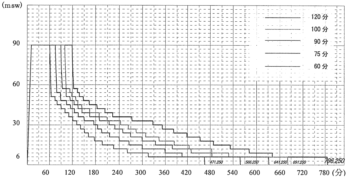
図2-26 ヘリオックス減圧過程図 (90msw)-まとめ
