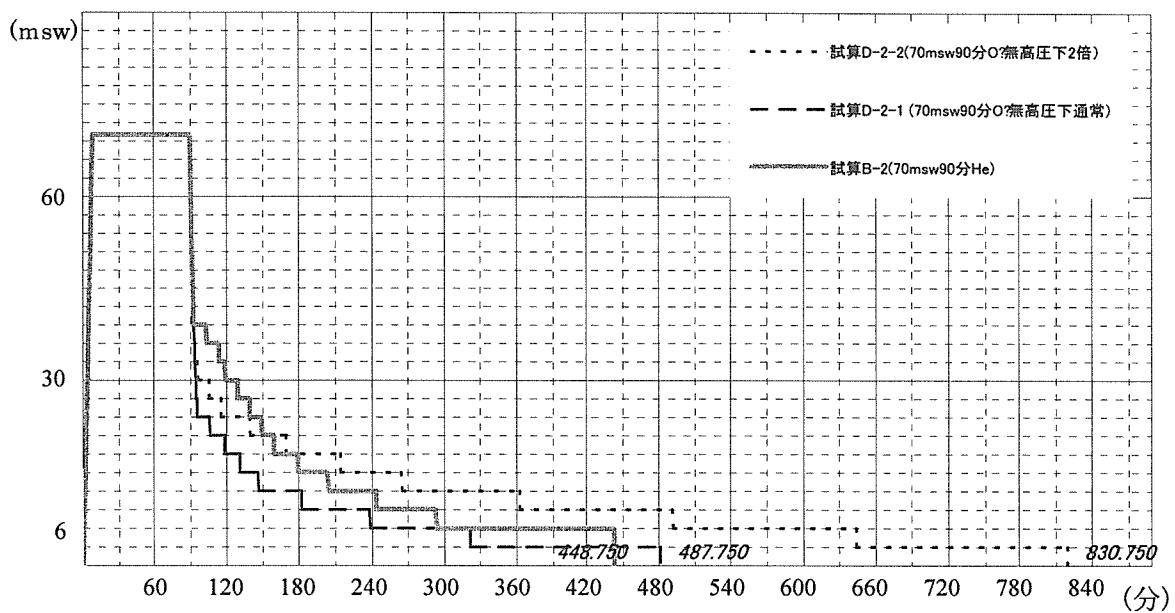
図2-46 緊急時空気（酸素吸入不能）減圧過程図(70msw,90分)
