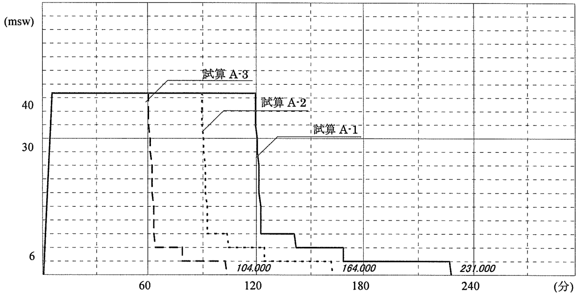
図2-51 ナイトロックス減圧過程図(40msw)-まとめ
