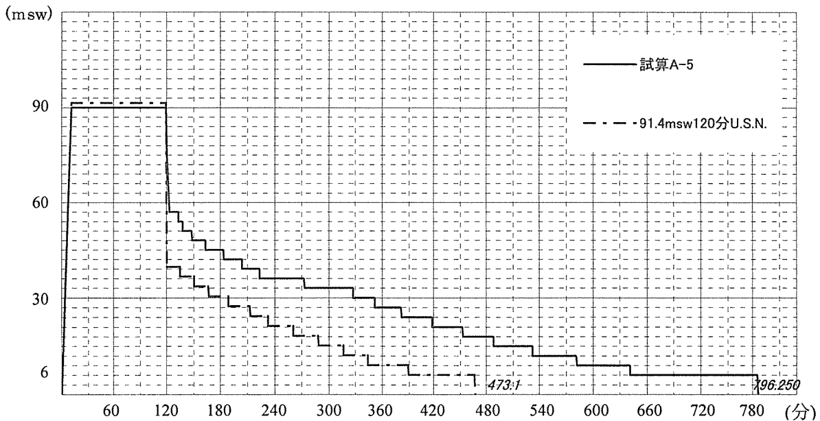
図2-27 ヘリオックス減圧過程図(90msw,120分)
