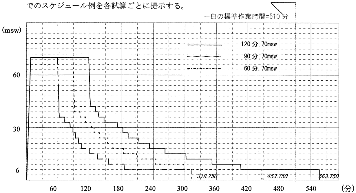
図2-34 ヘリオックス減圧過程図(70msw)-まとめ
