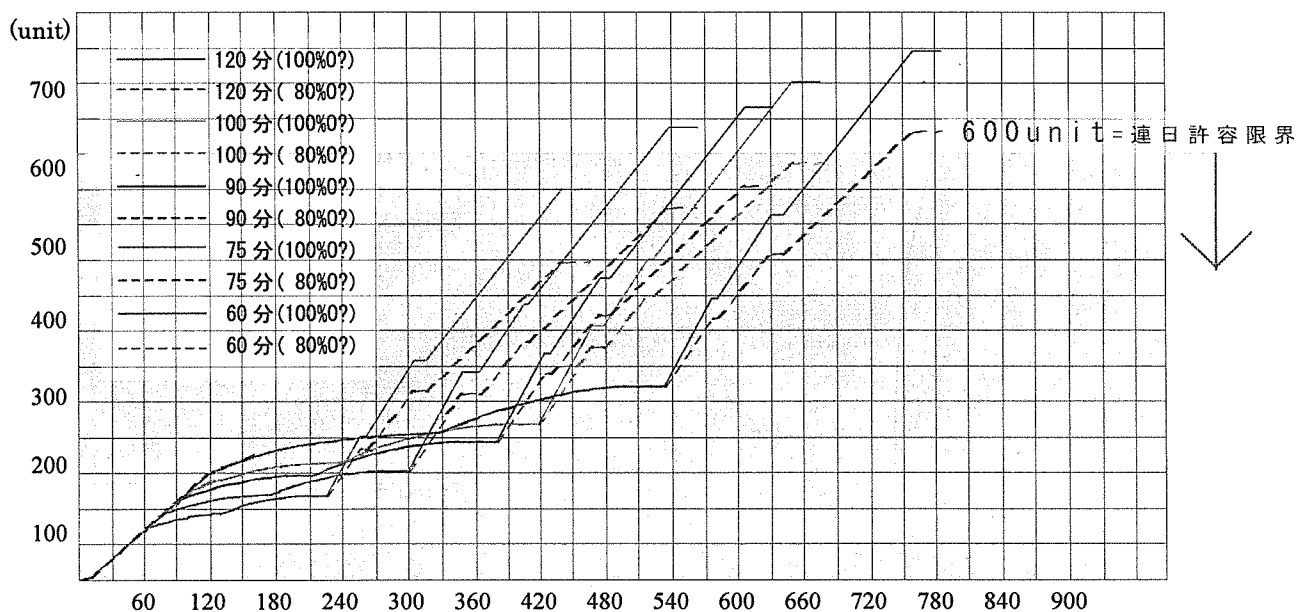
図2-28 OTU増減 (90msw)-まとめ
