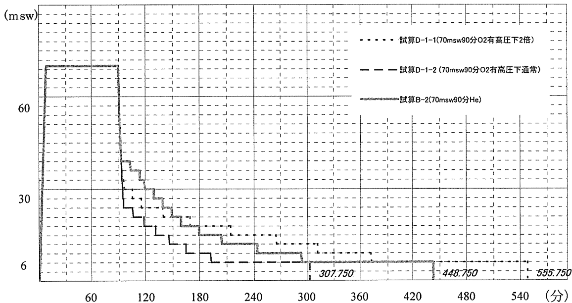
図2-45 緊急時空気（酸素吸入可能）減圧過程図(70msw,90分)
