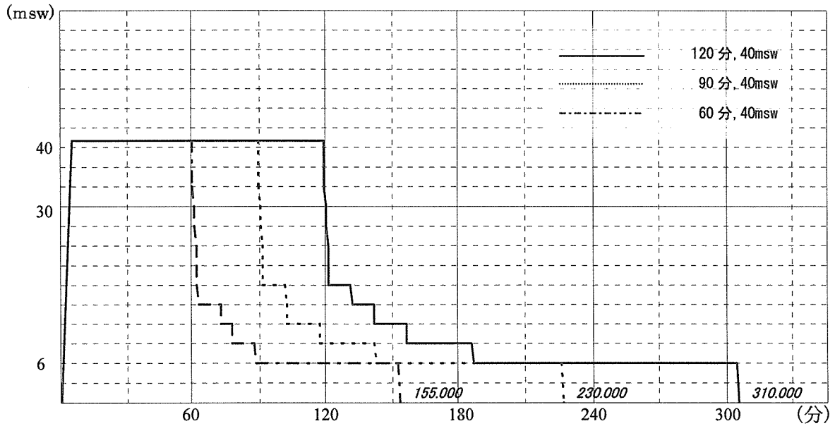
図2-40 ヘリオックス減圧過程図(40msw) -まとめ
