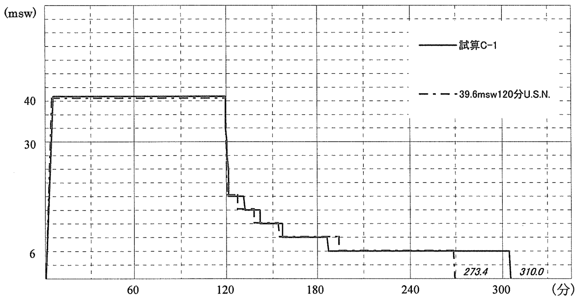
図2-41 ヘリオックス減圧過程図(40msw,120分)
