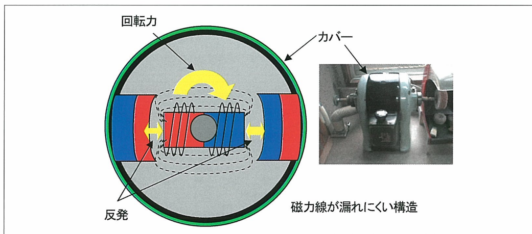
図80 回転型モータの模式図
