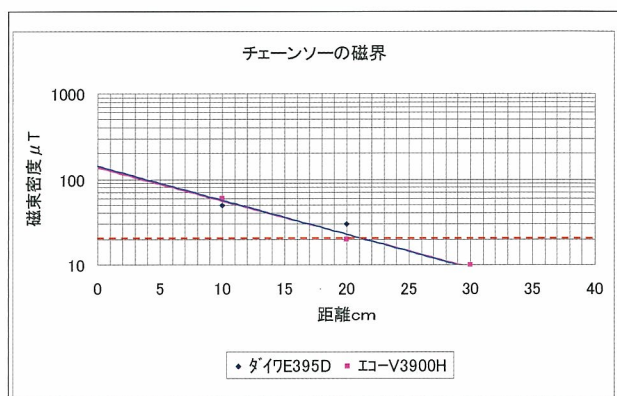
図85 チェーンソー
