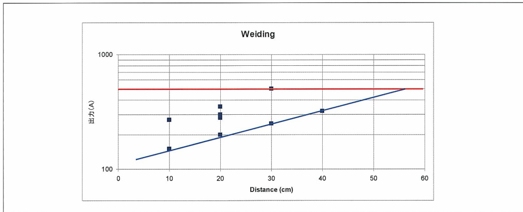
図 77 溶接電流と影響の距離
