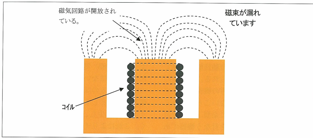
図82 脱磁気装置の模式図
