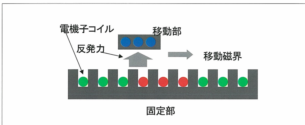
図81 リニアモータの模式図
