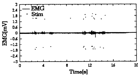
図 13: 歩行中の筋電図を用いて刺激の制御を行なった結果 (前頸骨筋)
