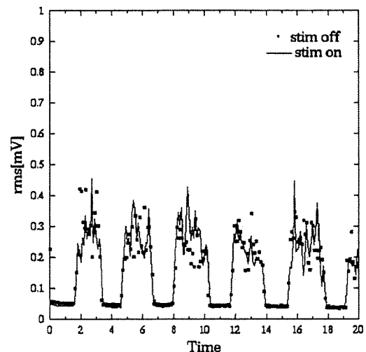
図9 C タイプに電極を配置した場合
