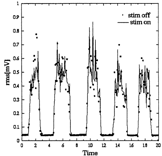
図8 B タイプに電極を配置した場合
