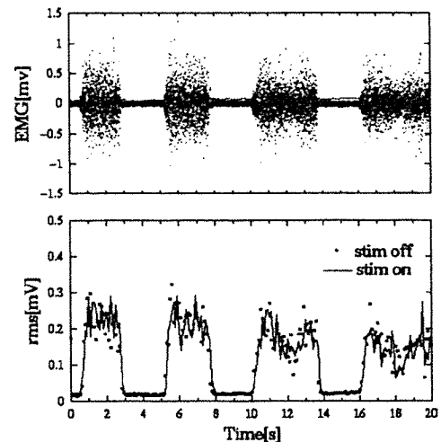
図 6: 刺激のある場合と無い場合での筋電図の比較 A タイプに電極を配置した場合
