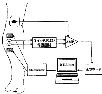
図 1 本研究における制御方式の概略図
