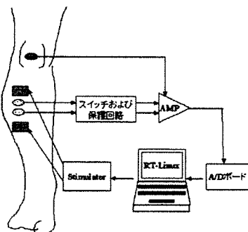
図 1: 本研究における制御方式の概略図
