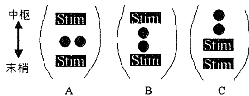
図7 刺激用電極と計測用電極の配置について 刺激用電極と計測用電極の配置について A,B,C の 3 通りについて実験を行ないいずれの配置が最も良いかについて比較を行なった。
