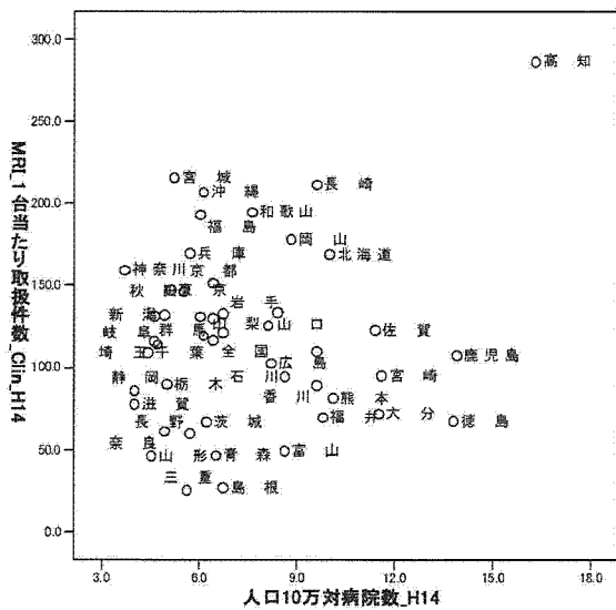
図 3.25: MRI 10万人当たり病院数×診療所1台当たり件数
