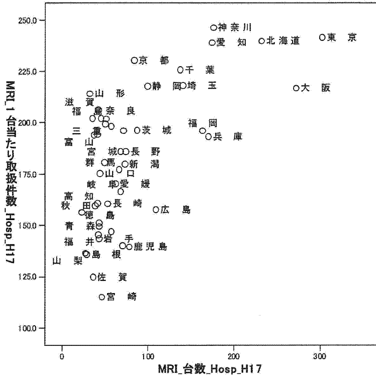
図 3.41: MRI 病院台数×病院1台当たり件数
