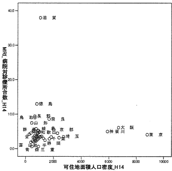
図 3.31: MRI 可住地面積人口密度×病院対診療所台数
