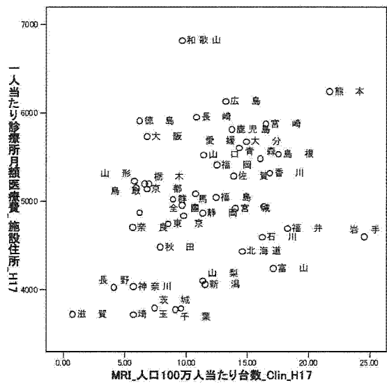
図 3.58: MRI 100万人あたり診療所台数×一人当たり診療所医療費
