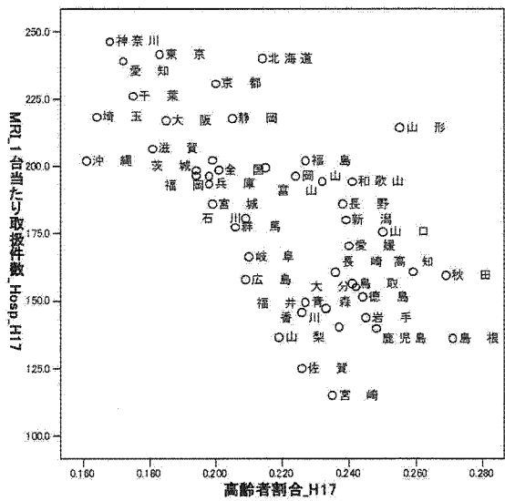
図 3.50: MRI 高齢者割合×病院1台
