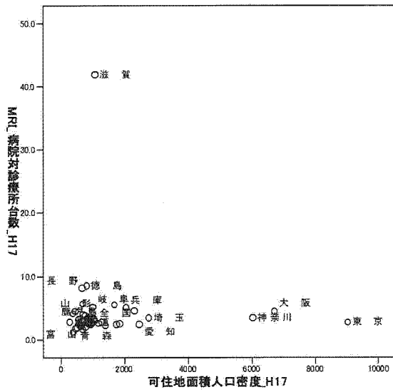
図 3.71: MRI 可住地面積人口密度×病院
