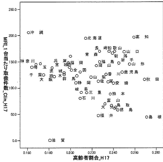
図 3.64: MRI 高齢者割合×診療所1台当たり件数
