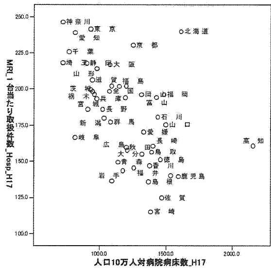
図 3.52: MRI 10 万人当たり病床数×病院 1 台あたり件数
