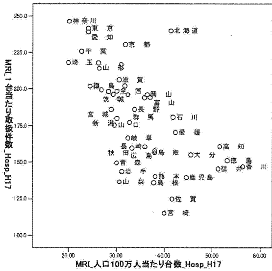
図 3.43: MRI 100 万人当たり病院台数×病院 1 台あたり件数
