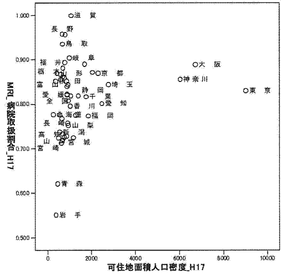
図 3.72: MRI 可住地面積人口密度×病院取割合
