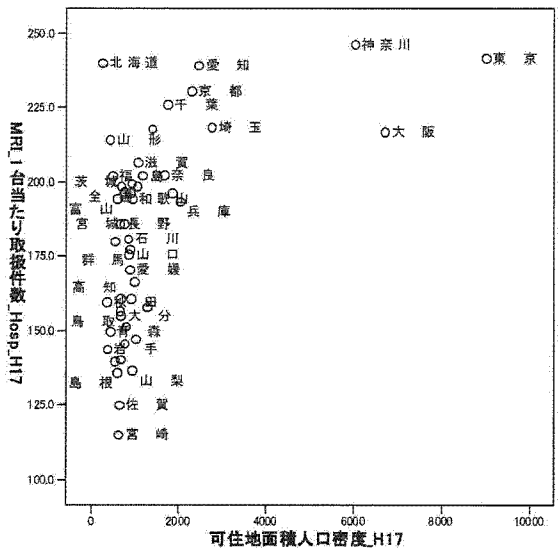
図 3.46: MRI 可住地面積人口密度×病院 1 台あたり件数
