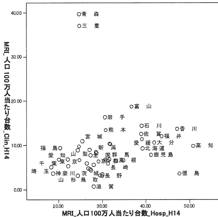
図 3.28: MRI 100万人あたり病院台数×100万人あたり診療所台数
