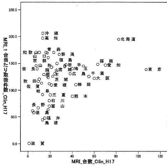
図 3.55: MRI 診療所台数×診療所1台当たり件数
