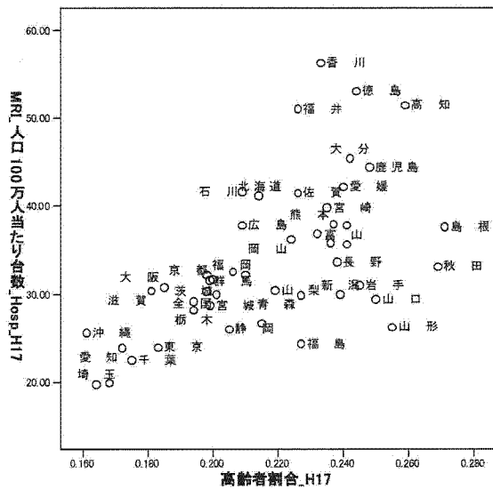
図 3.49: MRI 高齢者割合×100万人
