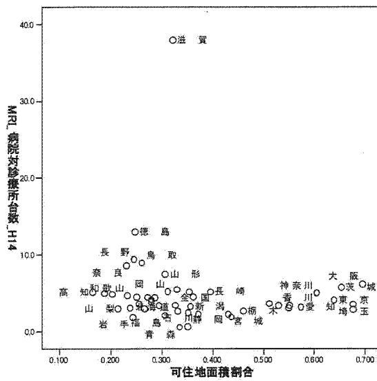
図 3.33: MRI 可住地面積割合×病院対診療所台数
