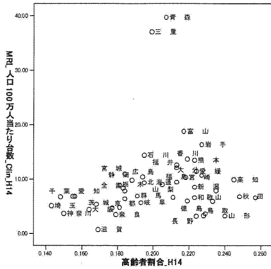
図 3.23: MRI 高齢者割合×100万人当たり診療所台数
