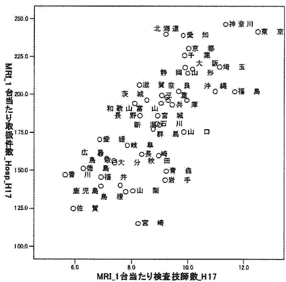
図 3.54: MRI 病院 1 台あたり技師数×病 院 1 台あたり件数
