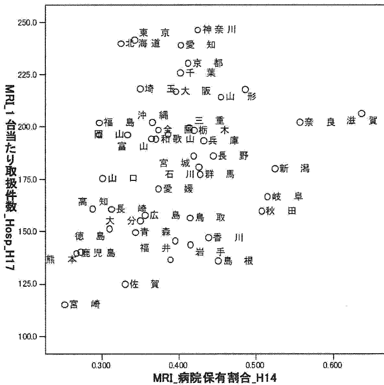
図 3.42: MRI 病院保有割合×病院1台当たり件数
