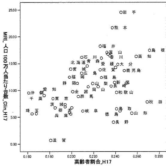
図 3.63: MRI 高齢者割合×100万人当たり診療所台数
