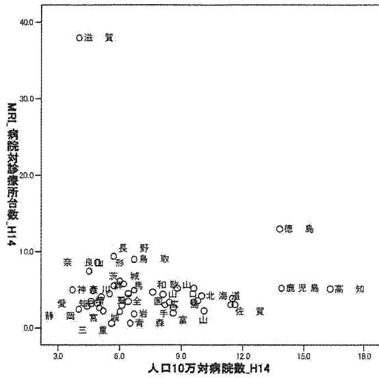
図 3.37: MRI 10 万人当たり病院数×病院対診療所台数
