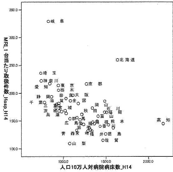
図 3.12: MRI 10 万人当たり病床数×病院 1 台当たり件数
