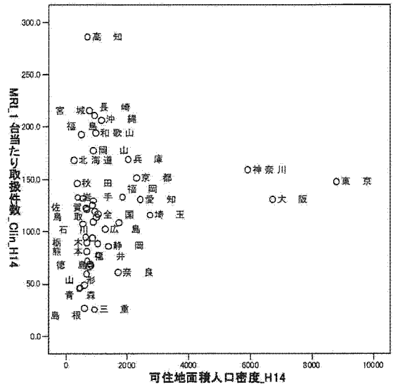
図 3.20: MRI 可住地面積人口密度×診療所1台当たり件数
