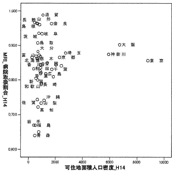
図 3.32: MRI 可住地面積人口密度×病院取割割合
