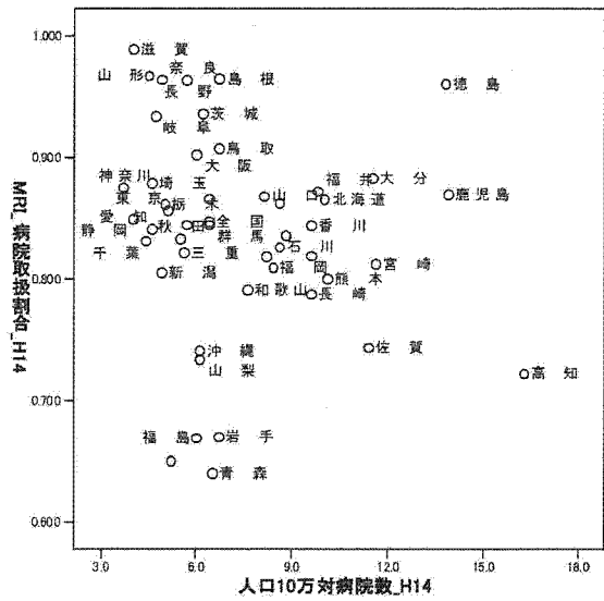
図 3.38: MRI 10 万人当たり病院数×病院取扱割合
