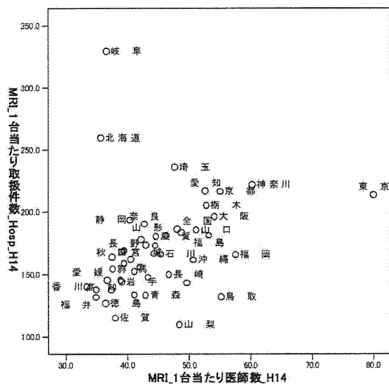
図 3.13: MRI 病院 1 台当たり医師数×病 院 1 台当たり件数
