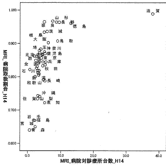
図 3.29: MRI 病院対診療所台数×病院取割割合
