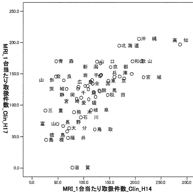
図 3.82: MRI 平成14年1台あたり件数×平成17年1台あたり件数
