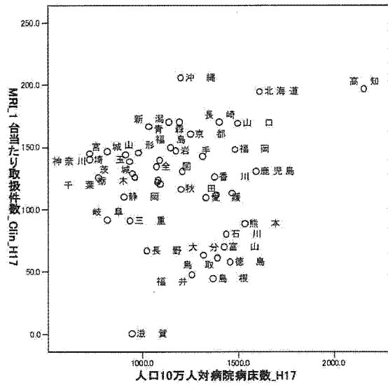
図 3.66: MRI 10万人当たり病床数×診療所1台当たり件数
