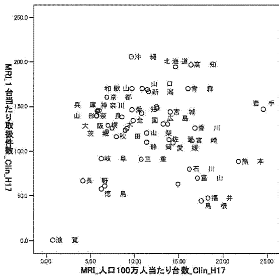
図 3.57: MRI 100万人あたり診療所台数×診療所1台当たり件数
