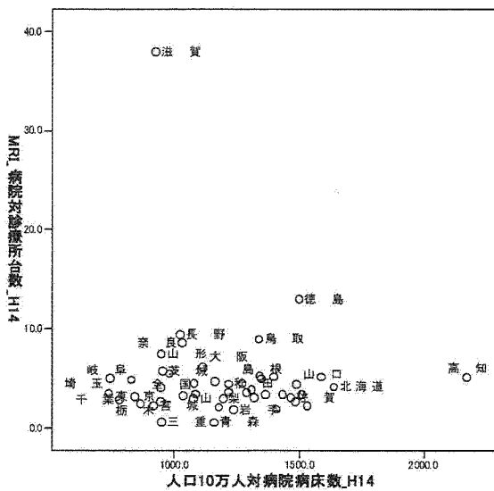
図 3.39: MRI 10 万人当たり病床数×病院対診療所台数
