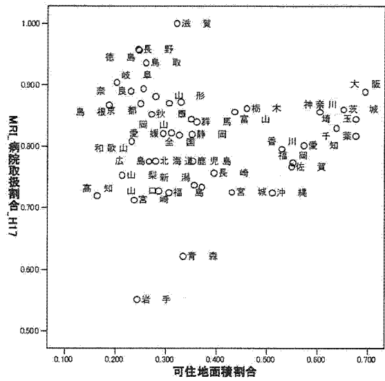
図 3.74: MRI 可住地面積割合×病院取扱割合
