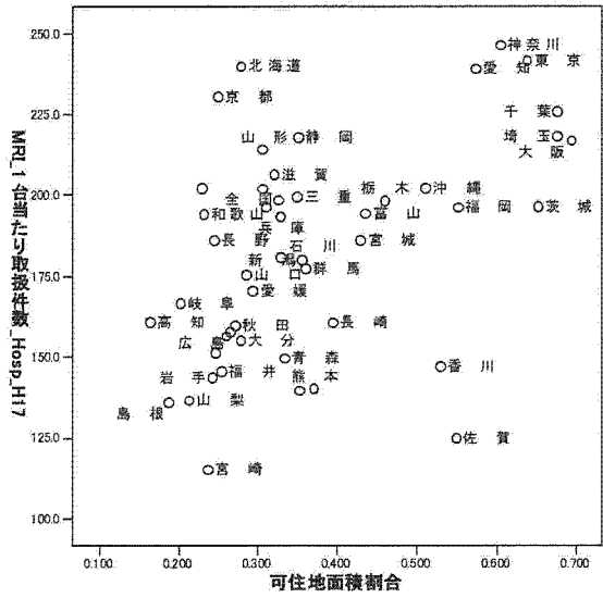
図 3.48: MRI 可住地面積割合×病院1台
