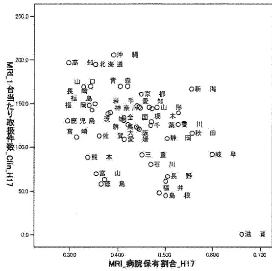
図 3.56: MRI 病院保有割合×診療所1台当たり件数
