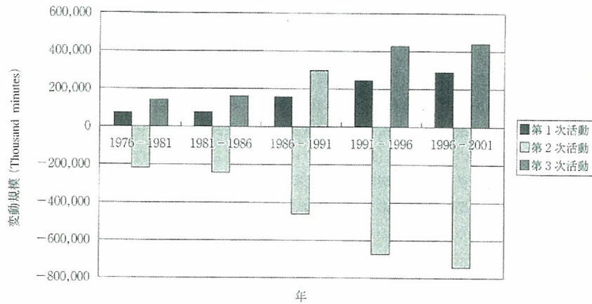
図12 高齢化効果
