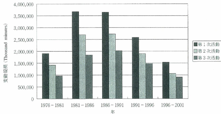
図10 成長効果
