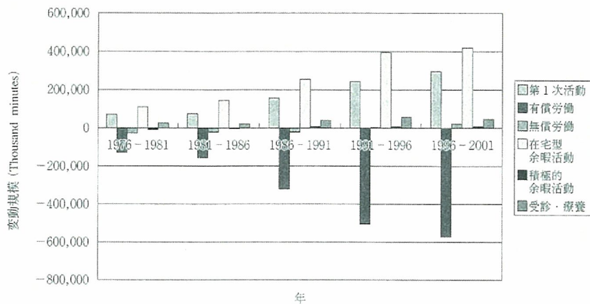
図13 高齢化効果
