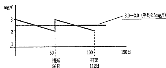
図 3-6 固体状防錆剤補充間隔(例)
