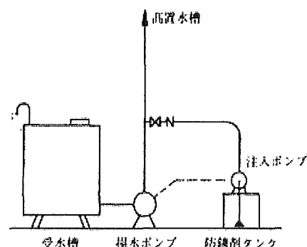
図 3-1 インターロック方式
