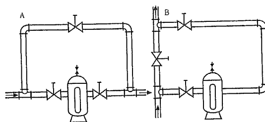
図 3-5 バイパス取り付け例
