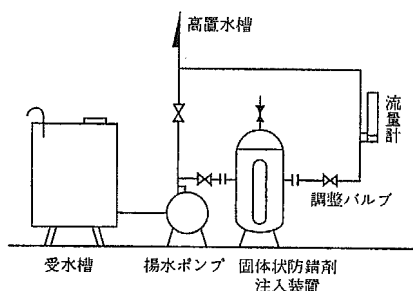
図 3-4 バイパス法(例)
