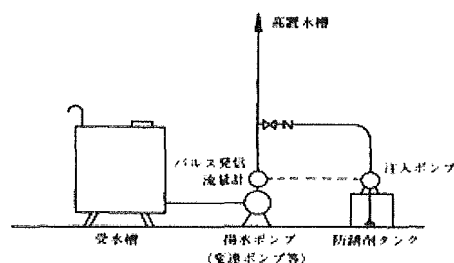
図 3-2 流量比例注入方式(例)
