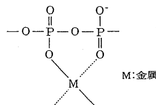
図 2-3 キレート結合
