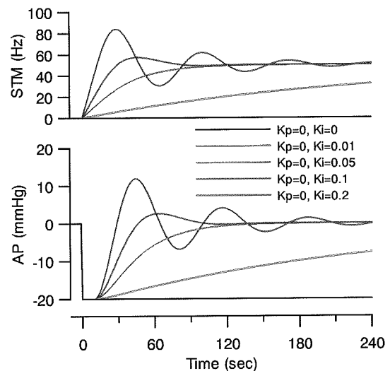
図C-5-1. K_p=0 の場合
