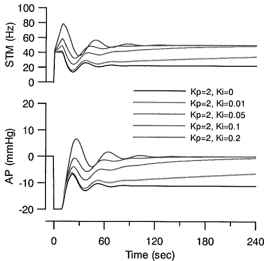
図C-5-2. K_p=2 の場合
