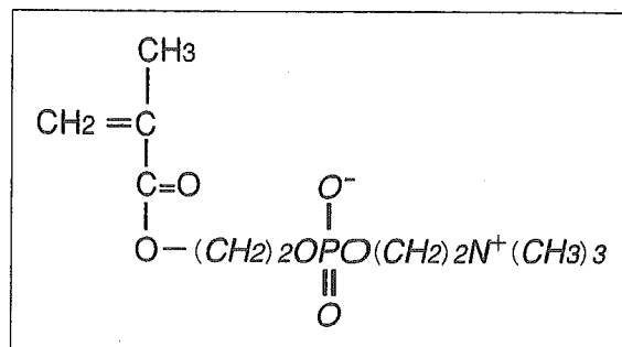
図1 MPCの構造
