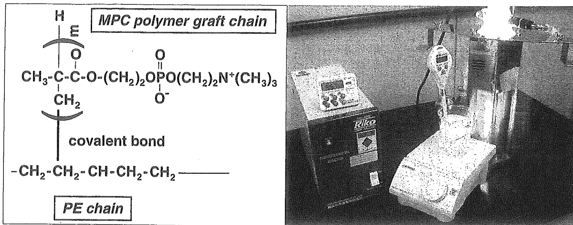
図1 MPCポリマー処理 紫外線を用いてMPCポリマー鎖とPEの炭素原子同士に安定な共有結合をさせるもので、 ナノオーダーの表層のみの処理であり、基材であるPE自体には影響を及ぼさない。
