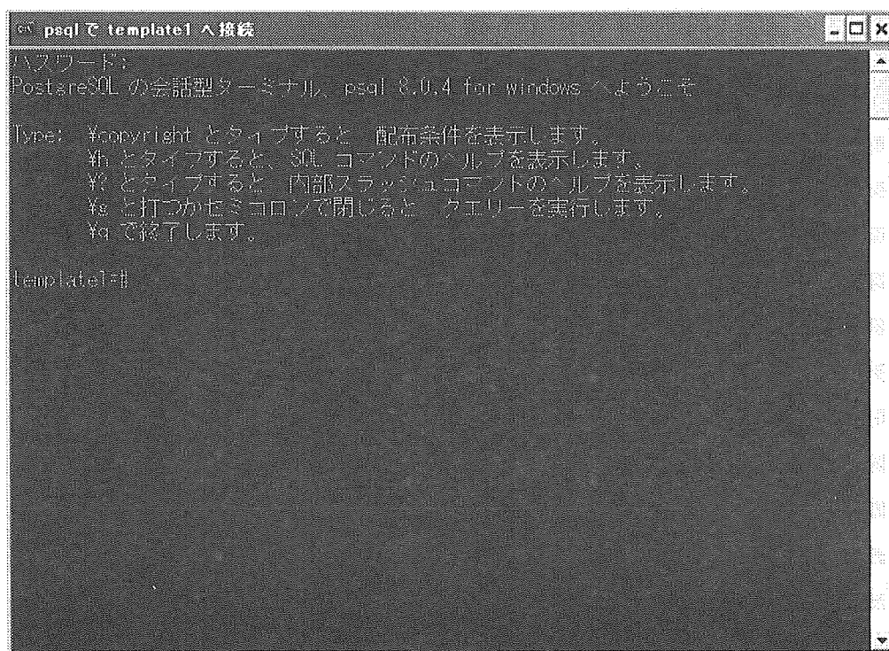
● 図4-1-2 「psql」画面
