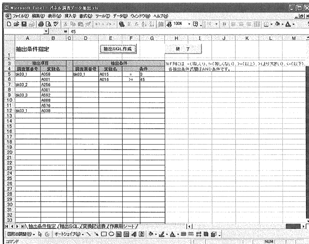
● 図 2 - 1 抽出条件指定画面
