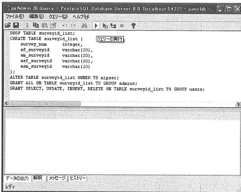
● 図 2-3-4 [pgAdminIII Query] ウィンドウ クエリーの実行
