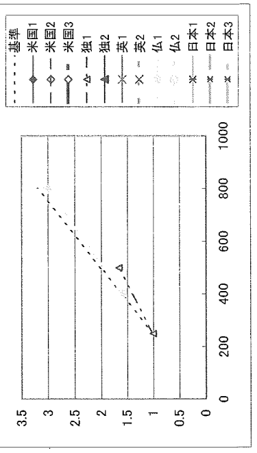
メカバジン
