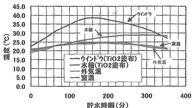
図11 アクアウインドウ貯水温の経時変化(晴天時)
