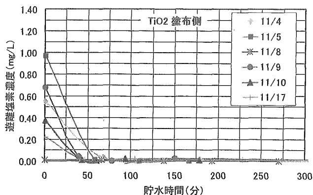
図13 アクアウインドウ貯水の遊離塩素濃度の経時変化(晴天時、塗布側)
