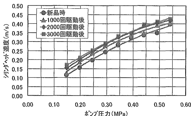
図 8 シリンダ駆動回数がシリンダヘッド速度に与える影響(アクアシリンダの耐久性)
