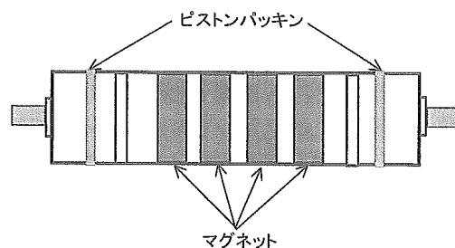
図5 シリンダ内部移動子の概略
