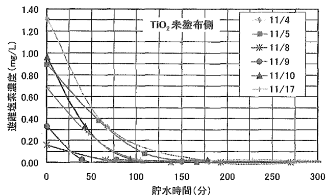
図14 アクアウインドウ貯水の遊離塩素濃度の経時変化(晴天時、未塗布側)
