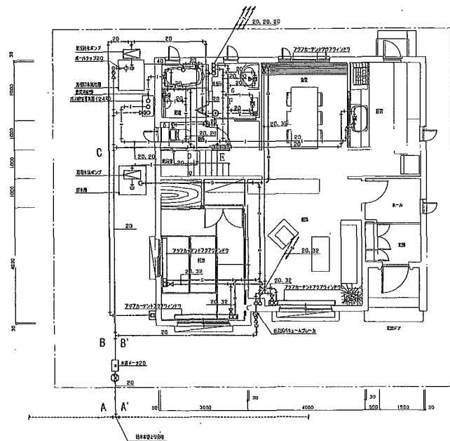
1階平面図
