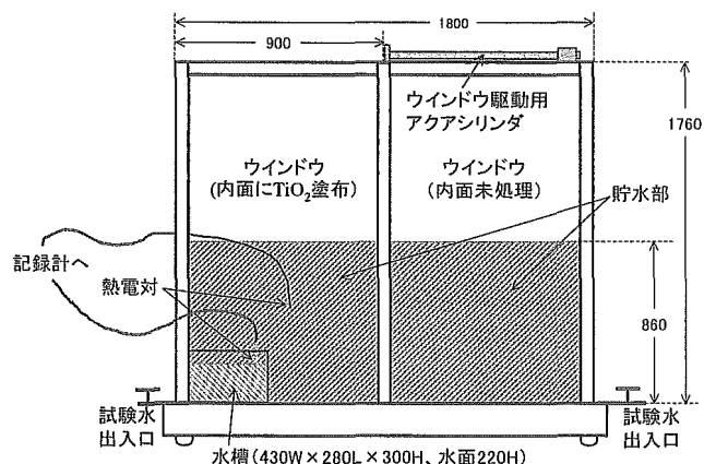
図10 アクアウィンドウプロト機の概略図
