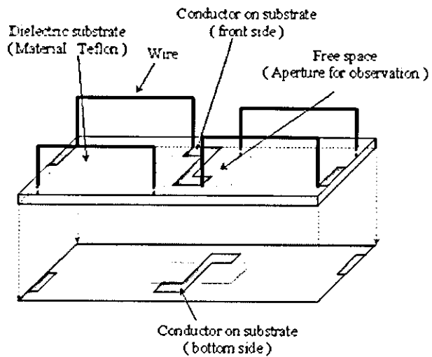
図1 8の字ループアンテナ概略図
