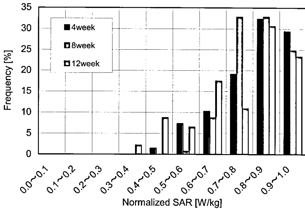
図 11 各週齢のラット標的組織内 SAR ヒストグラム
