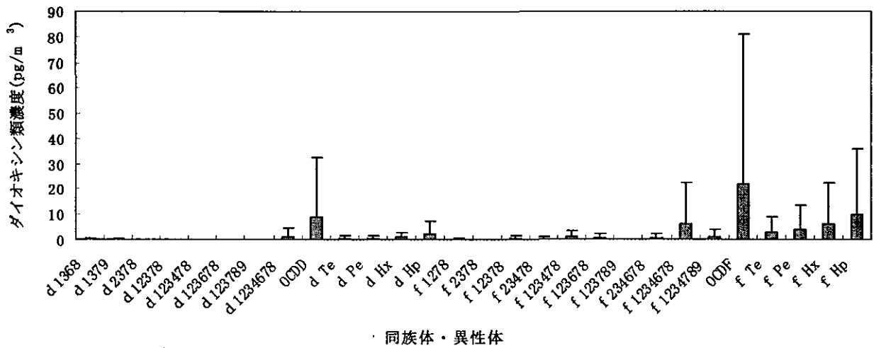
図5-1 気中塩素化ダイオキシン類(PCDD/PCDF)濃度の同族体・異性体分布(実測濃度)(RDF)
