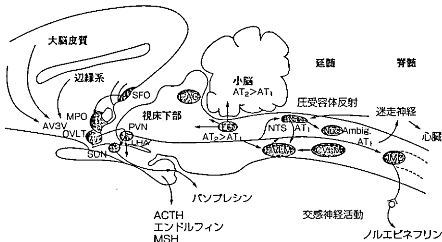
図② アンジオテンシンIIが循環調節に関与するラット脳内部位と受容体サブタイプ AV3V: 第三脳室前腹側部, SFO: 脳弓下器官, MPO: 内側視索前核, OVLTL: 終板器官, PVN: 室傍核, LHA: 外側視床下部, SON: 視索上核, PAG: 中脳水道周辺灰白質, LC: 青斑核, NTS: 弧束核, RVLM: 吻側延髄腹外側野, CVLM: 尾側延髄腹外側野, Nuc. Ambig.: 疑核, IML: 中間質外側核。
