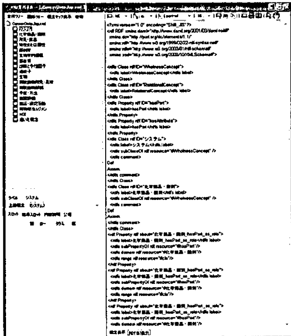
図1. オントロジーエディタ「製造」を用いたがん化学薬品・薬剤オントロジの日本語化.
