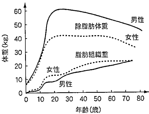
図3 加齢と脂肪組織重, 除脂肪体重の変化 (秦 霞哉: 高齢者の栄養, 日本老年医学会編, 老年医学テキスト, 東京, メジカルビュー社, 74-82, 1997 より一部改変)
