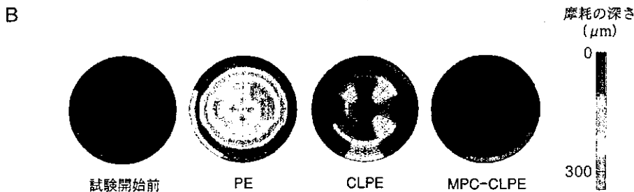
図 3 股関節シミュレーター試験の結果 [文献 15] を一部改変
