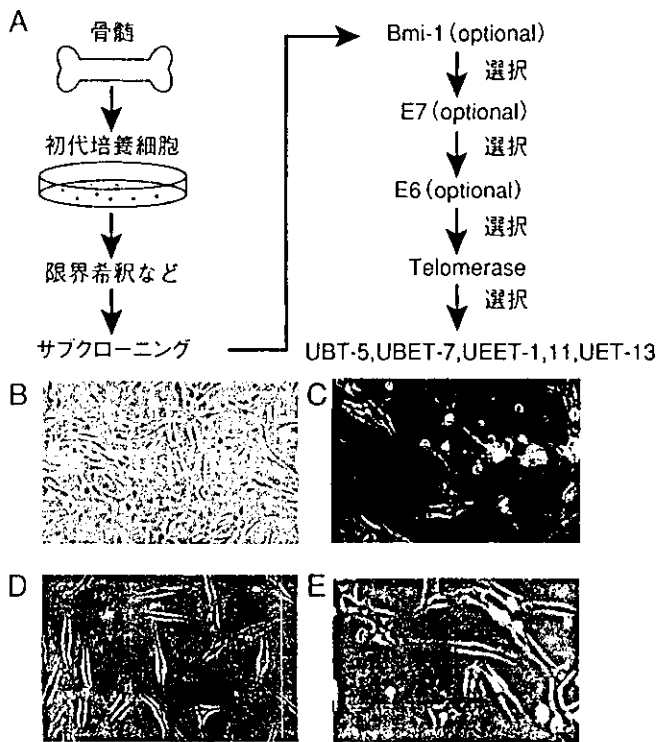
図3 ヒト骨髄間質細胞の寿命延長
