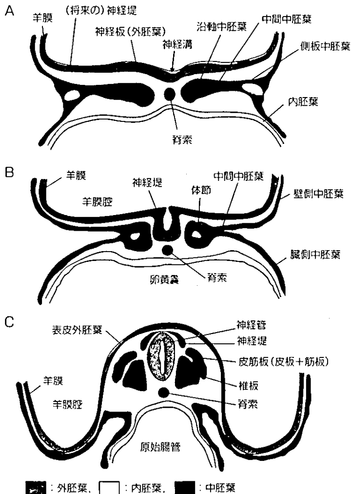
図1 体節の分化
