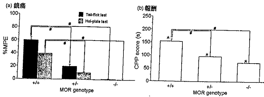
図1 野生型、ヘテロ型並びにホモ型の MOR-KO マウスにおけるブプレノルフィン (3.0 mg/kg, s.c) の作用 (a) ブプレノルフィンの鎮痛効果。ブプレノルフィン投与により、野生型 (+/+), ヘテロ型 (+/-) 並びにホモ型 (-/-) の MOR-KO マウスにおいて、Tail-flick 法 (■) および Hot-plate 法 (●) 共に %MPE に有意な変化を生じた。# 野生型マウスと比較して有意な差が見られる ( P < 0.05 ) (b) ブプレノルフィンの報酬効果。野生型 (+/+), ヘテロ型 (+/-) 並びにホモ型 (-/-) の MOR-KO マウスにおける CPP scores を示す。# 野生型マウスと比較して有意な差が見られる ( P < 0.05 ). n.s., 有意差無し。* ブプレノルフィンによる条件付けの前後で、条件付けした compartment における滞在時間が有意に変化している ( P < 0.05 )。
