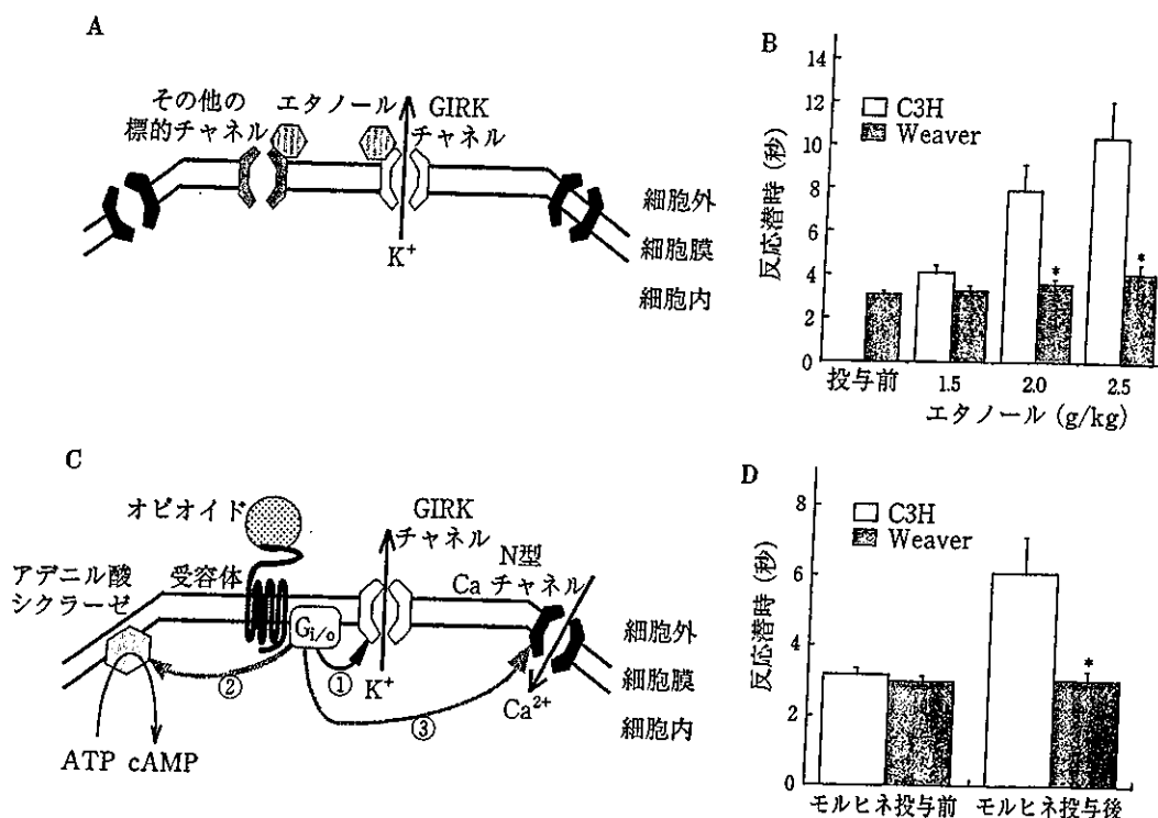
図1 エタノールとオピオイドのシグナル伝達経路でのGIRKチャンネルの役割 A: エタノール作用機序の模式図。エタノールはGIRKチャンネルや他の特定のイオンチャンネルに作用する。B: ウィーバーミュータントマウスとC3Hマウスでのエタノールの鎮痛効果(テールフリックテスト)。C: オピオイド作用機序の模式図。オピオイドはオピオイド受容体を活性化し、 G_{i/o} 蛋白質を介して、GIRKチャンネルを活性化(①)、アデニル酸シクラーゼを抑制(②)、カルシウムチャンネルを抑制(③)する。D: ウィーバーミュータントマウスとC3Hマウスでのオピオイドの鎮痛効果(テールフリックテスト)。
