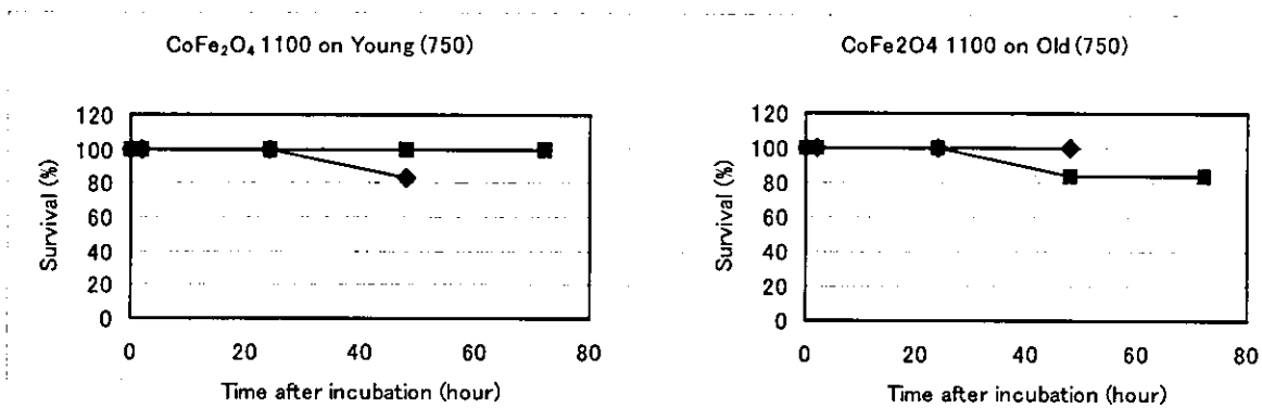
図 12 \text{CoFe}_2\text{O}_4 の細胞毒性テスト 3
