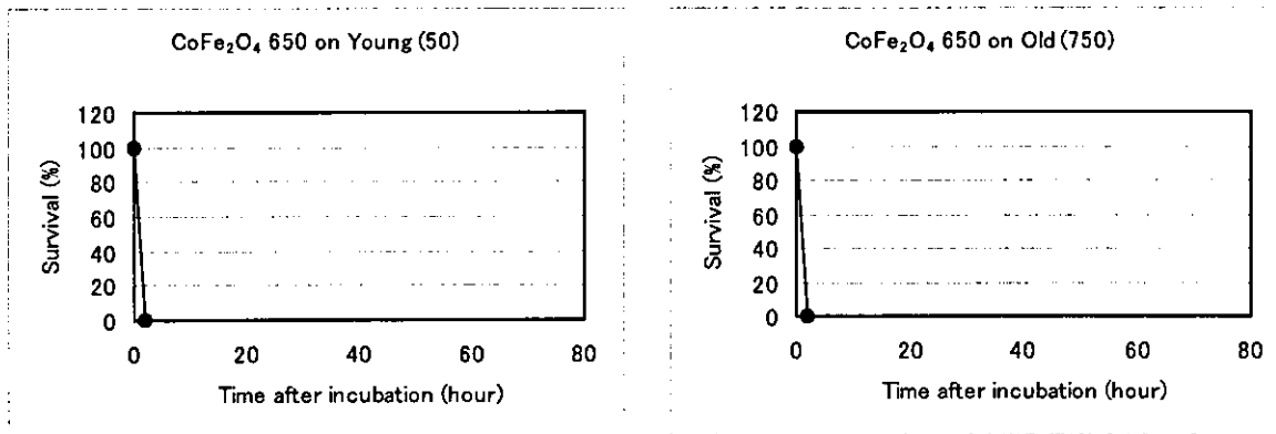
図10 CoFe 2 O 4 の細胞毒性テスト1
