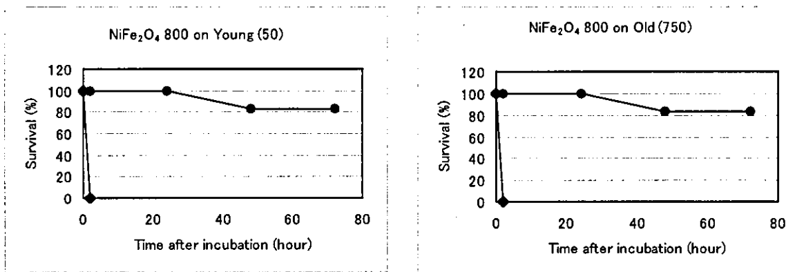
図9 NiFe 2 O 4 の細胞毒性テスト2
