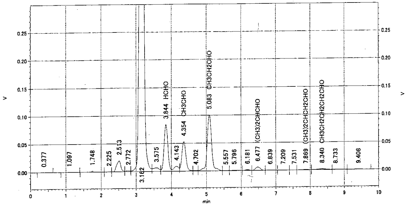
Ⅲ クロマトグラム⑦ アルデヒド類 (冬 個人)
