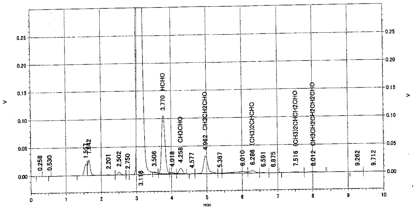
III クロマトグラム④ アルデヒド類 (夏 個人)
