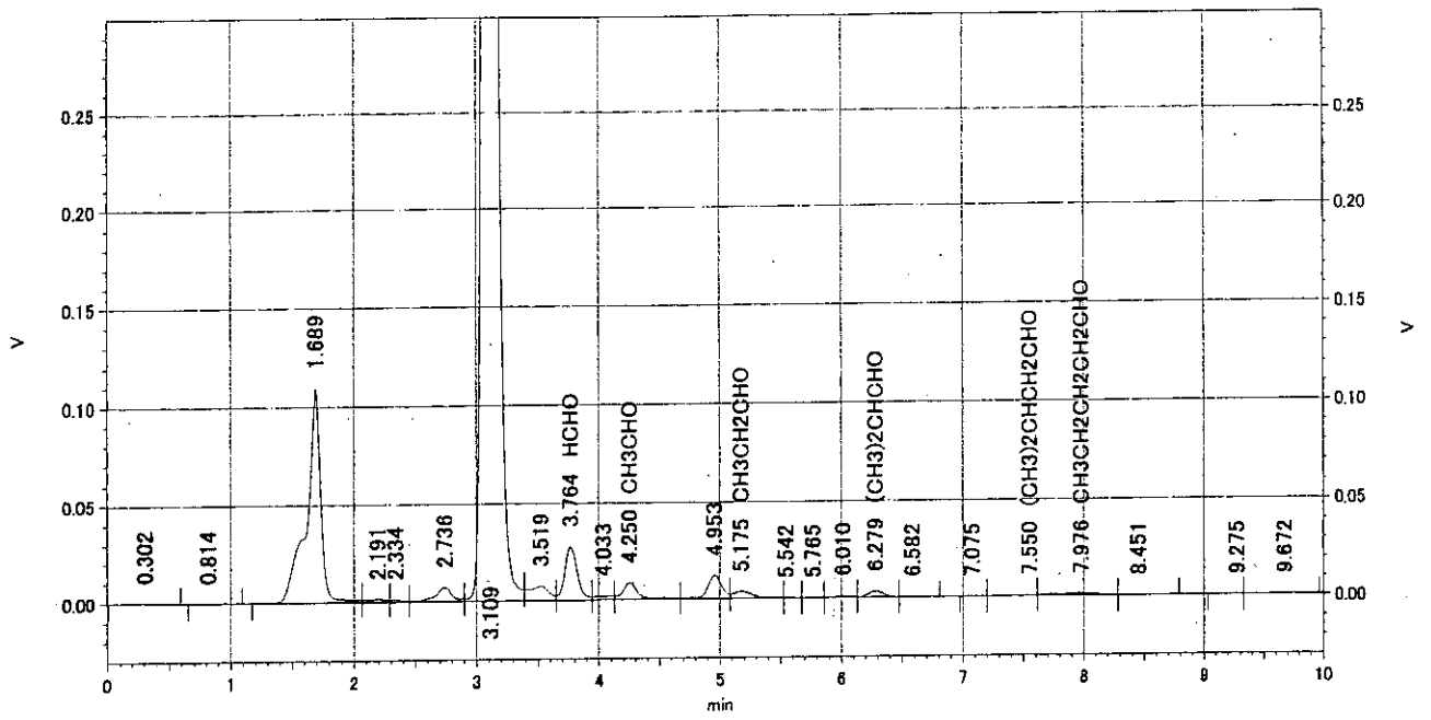
III クロマトグラム③ アルデヒド類 (夏 室外)
