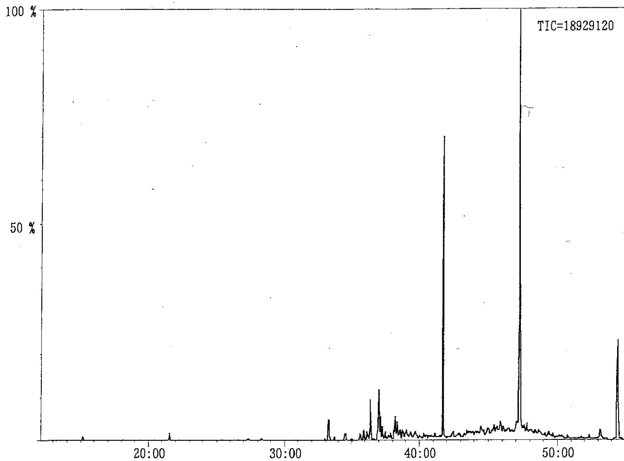
VI クロマトグラム② VOCs (低得点)
