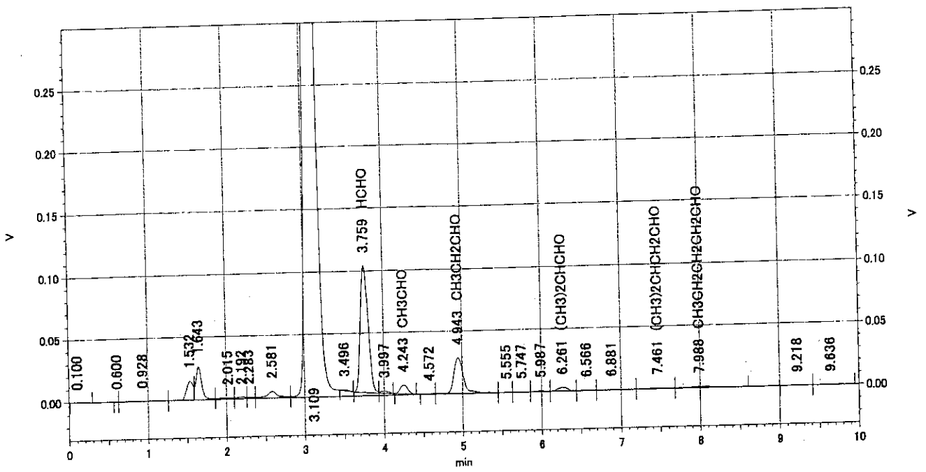
III クロマトグラム② アルデヒド類 (夏 居間)
