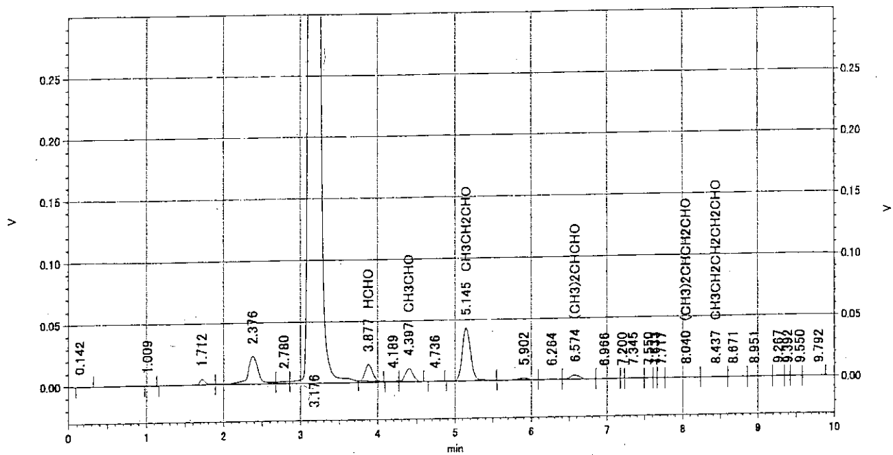
VI クロマトグラム⑤ アルデヒド類 (室外)
