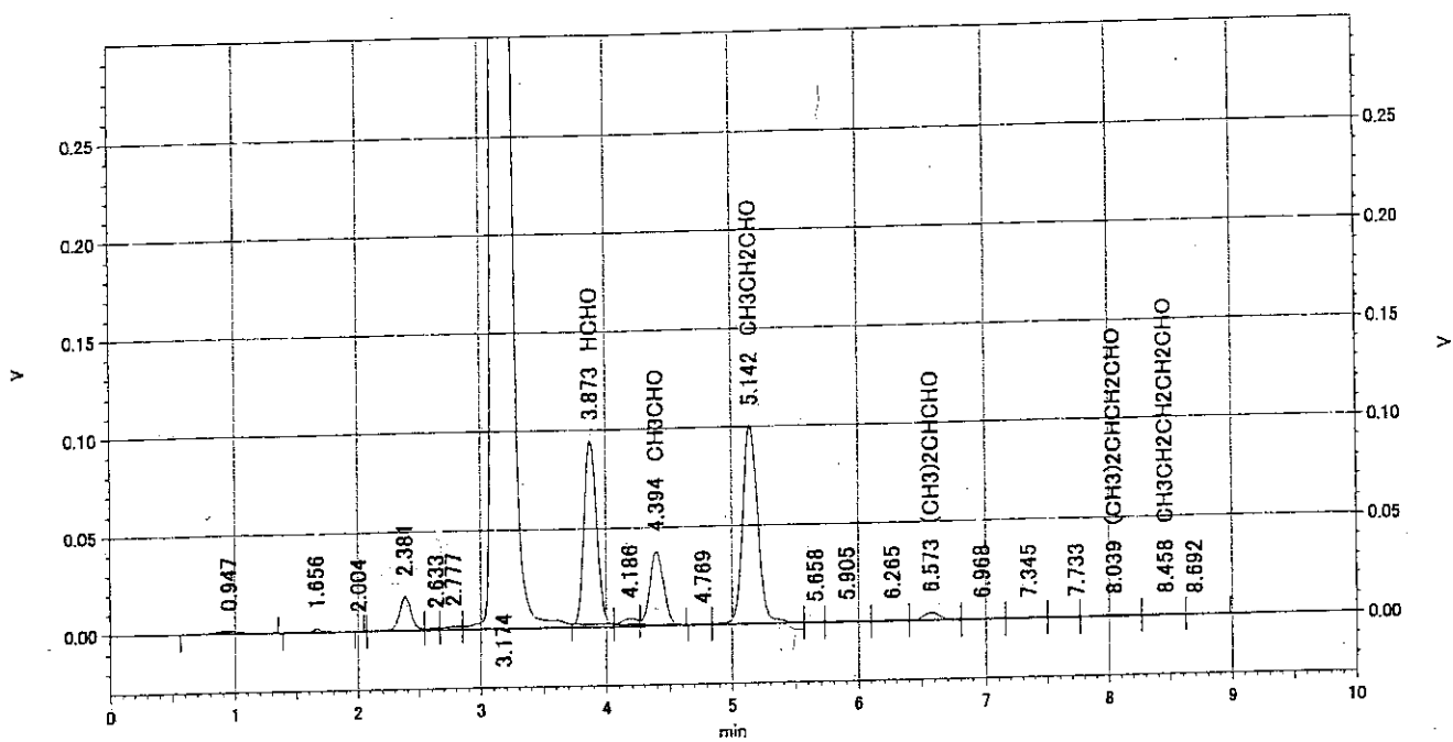
VI クロマトグラム④ アルデヒド類 (居間)
