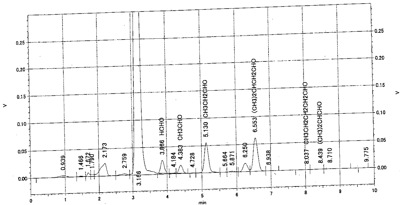
V クロマトグラム⑤ アルデヒド類 (室外)
