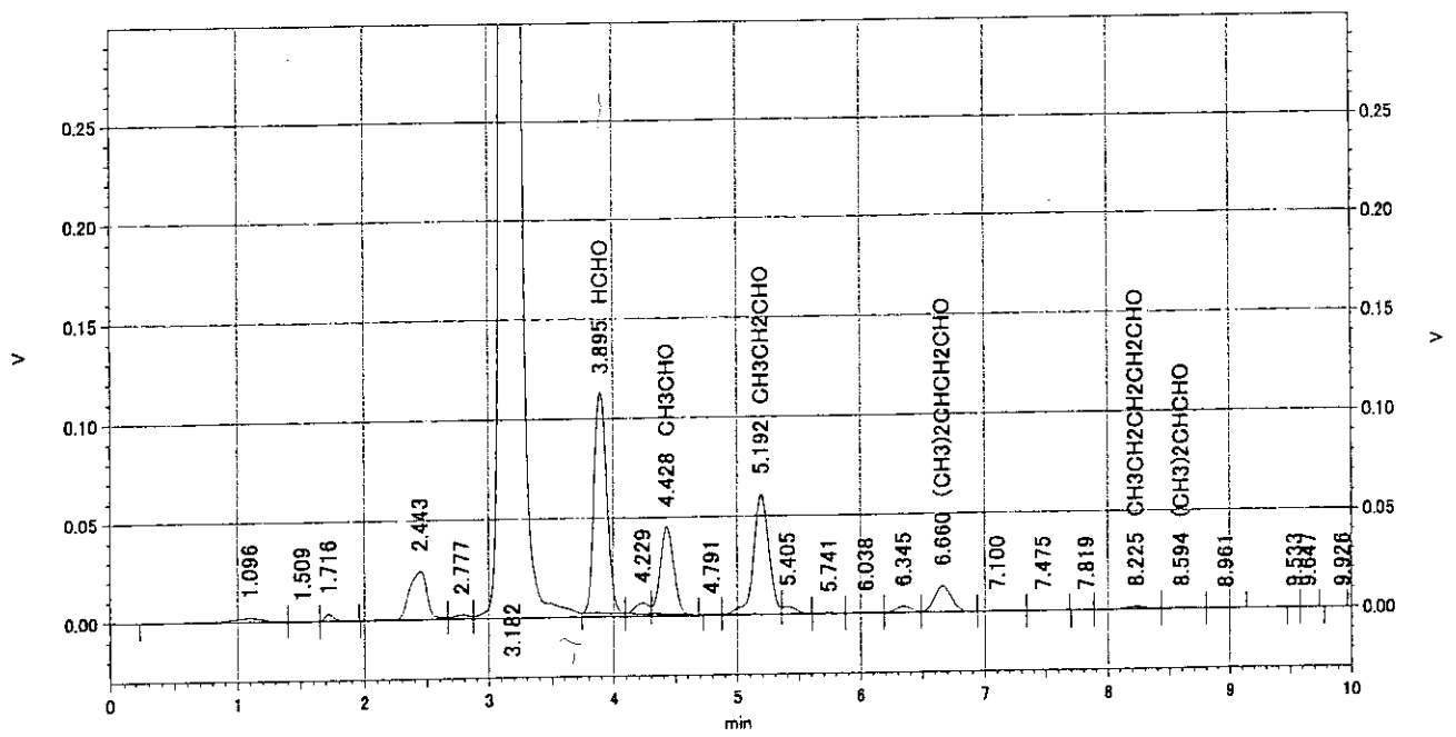
IV クロマトグラム② アルデヒド類 (個人C 1日目)
