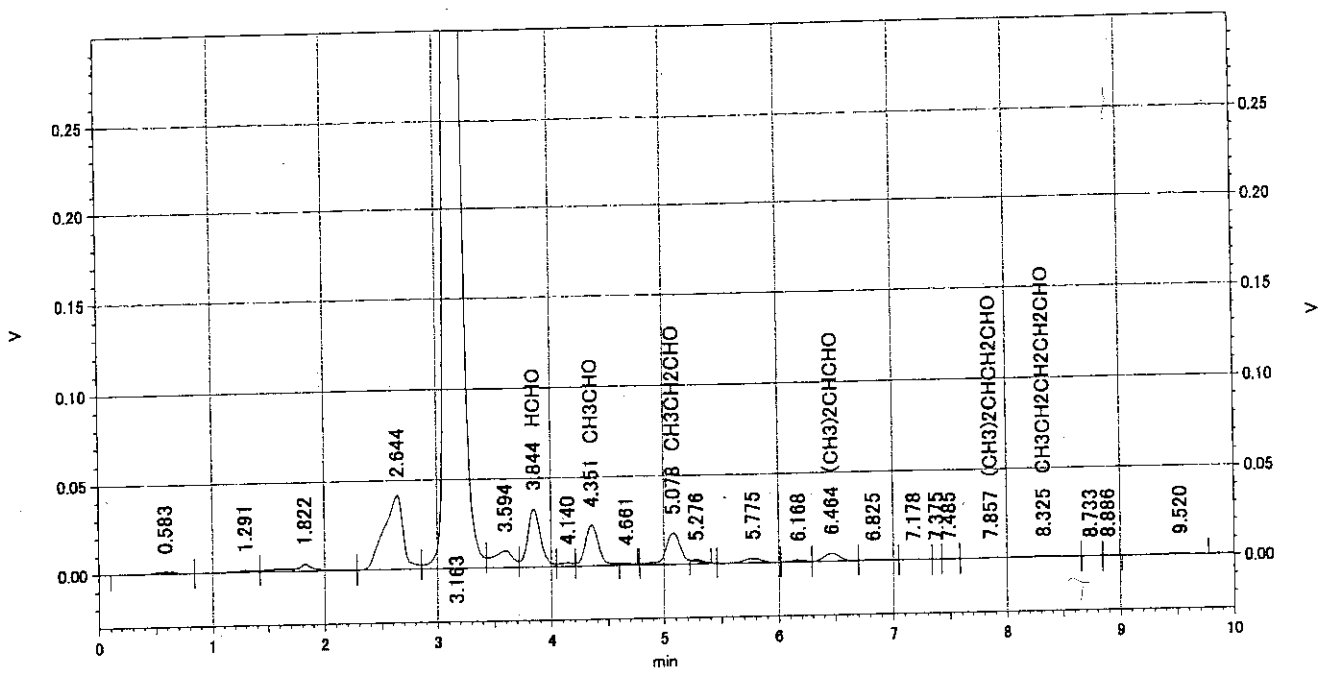
III クロマトグラム⑥ アルデヒド類 (冬 室外)
