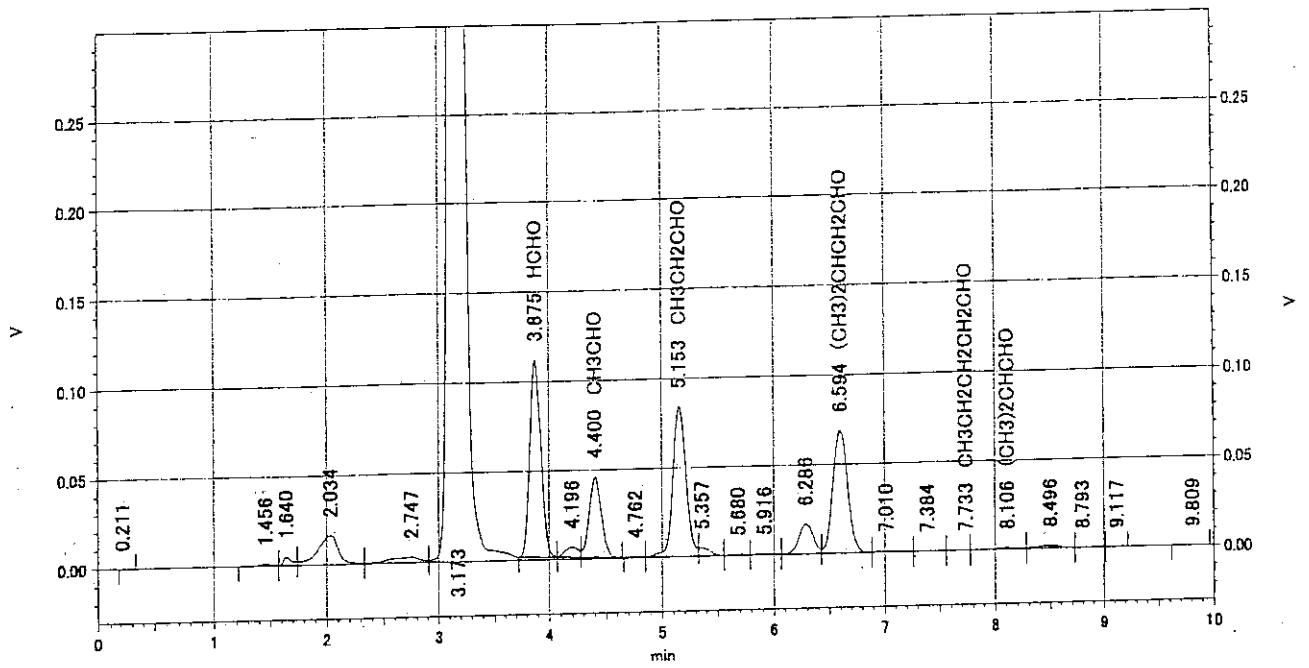
V クロマトグラム④ アルデヒド類 (居間)
