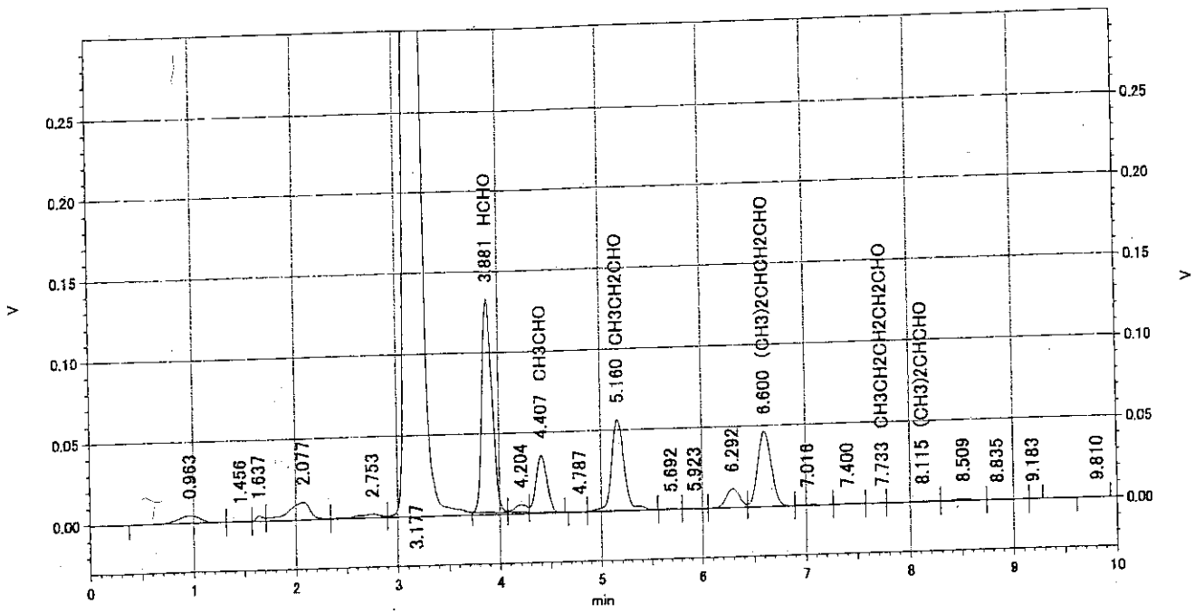
V クロマトグラム③ アルデヒド類 (子供部屋)
