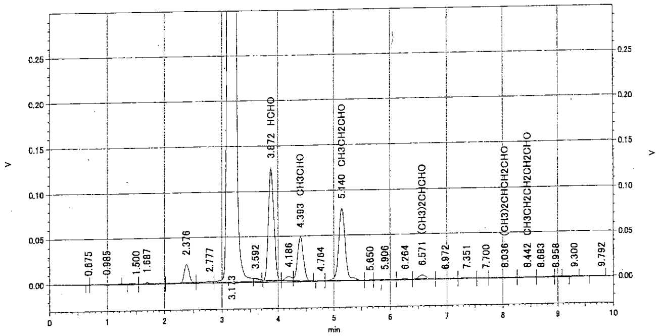
VI クロマトグラム③ アルデヒド類 (台所)
