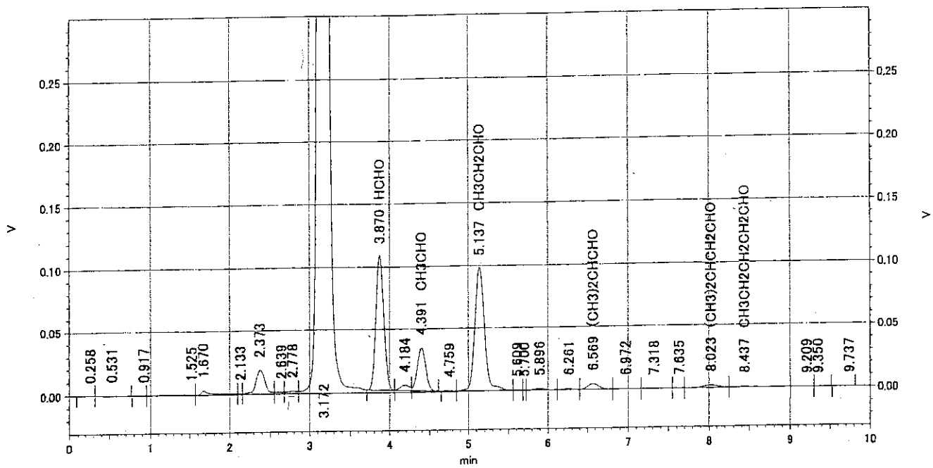
VI クロマトグラム⑥ アルデヒド類 (個人)
