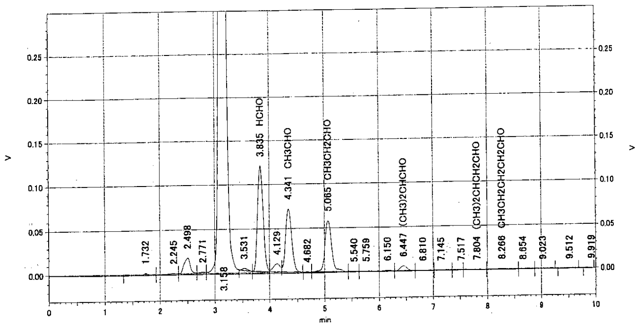
III クロマトグラム⑤ アルデヒド類 (冬・居間)
