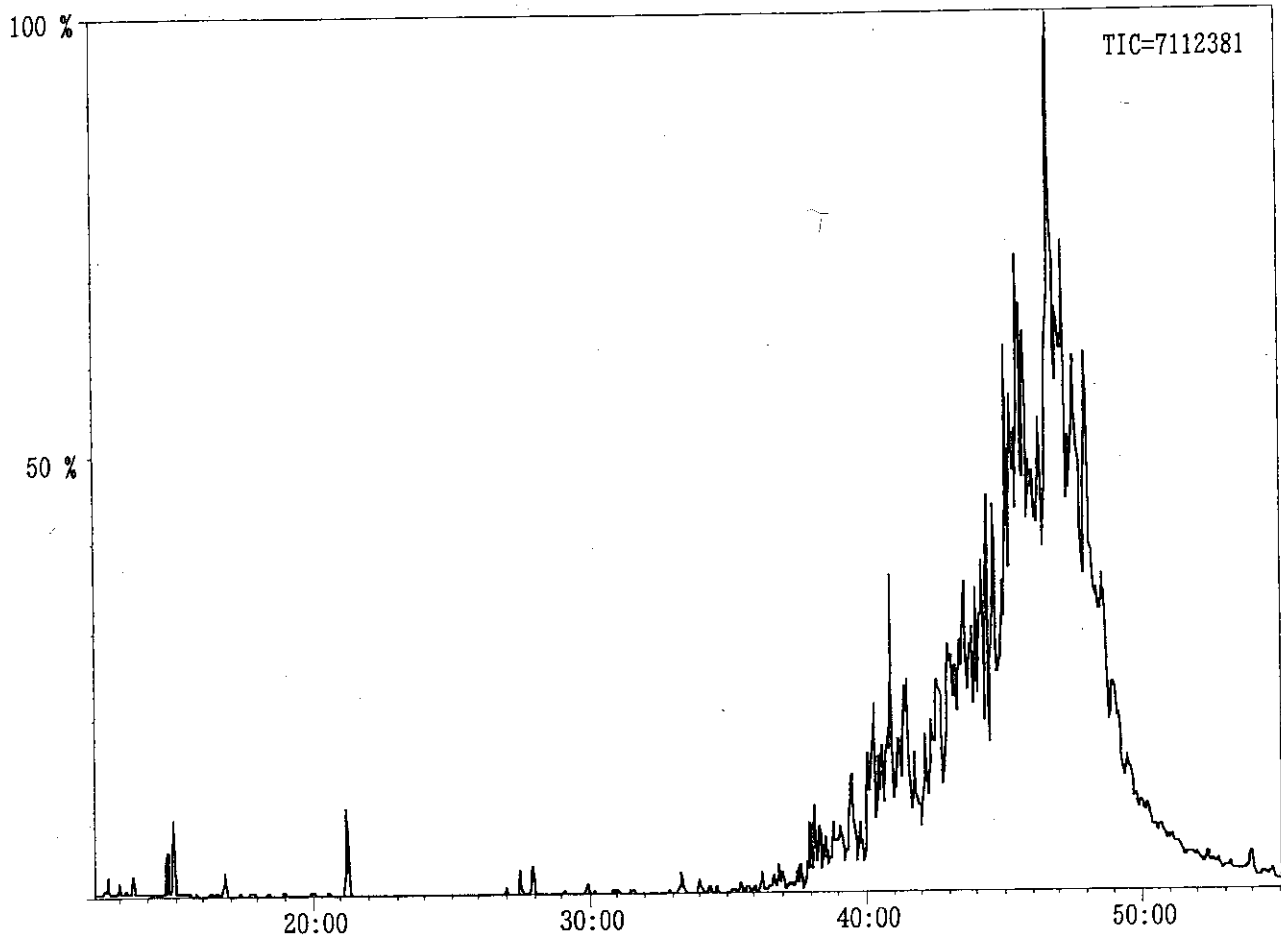
IV クロマトグラム① VOCs (個人 A 1 日目)
