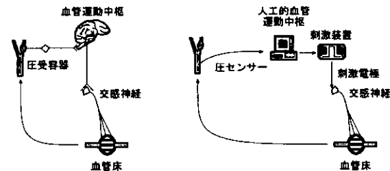
図A-6.生体固有の動脈圧反射とバイオニック動脈圧反射 (Pd、外乱)
