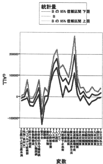
図C群 (cALL分析)
