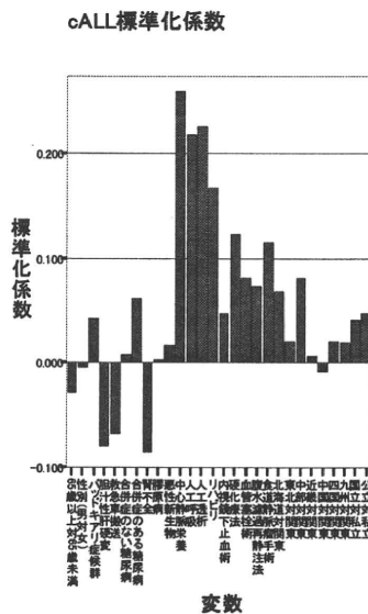
図C群 (cALL分析)
