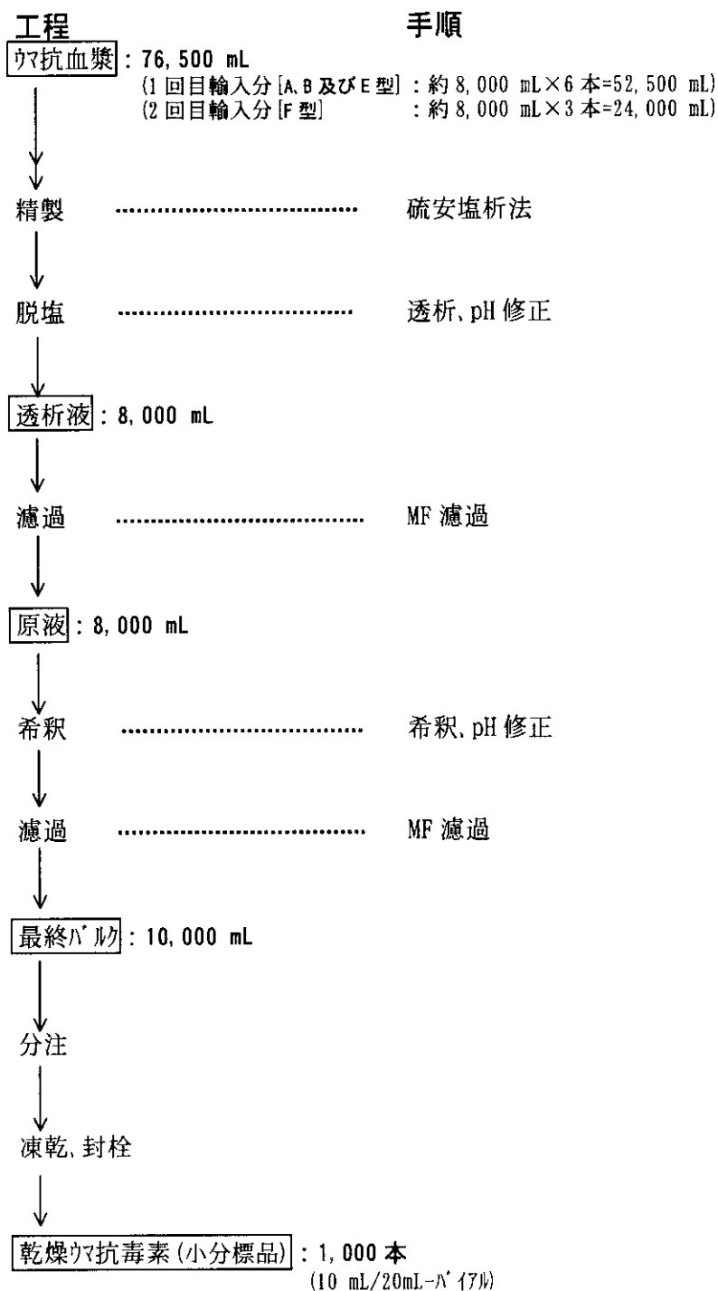
【図：ウマ抗血漿からの乾燥ウマ抗毒素の製造工程図】
