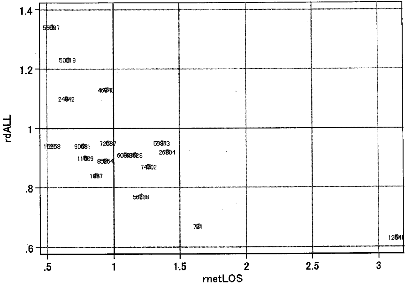
0600503x030x1x-density
