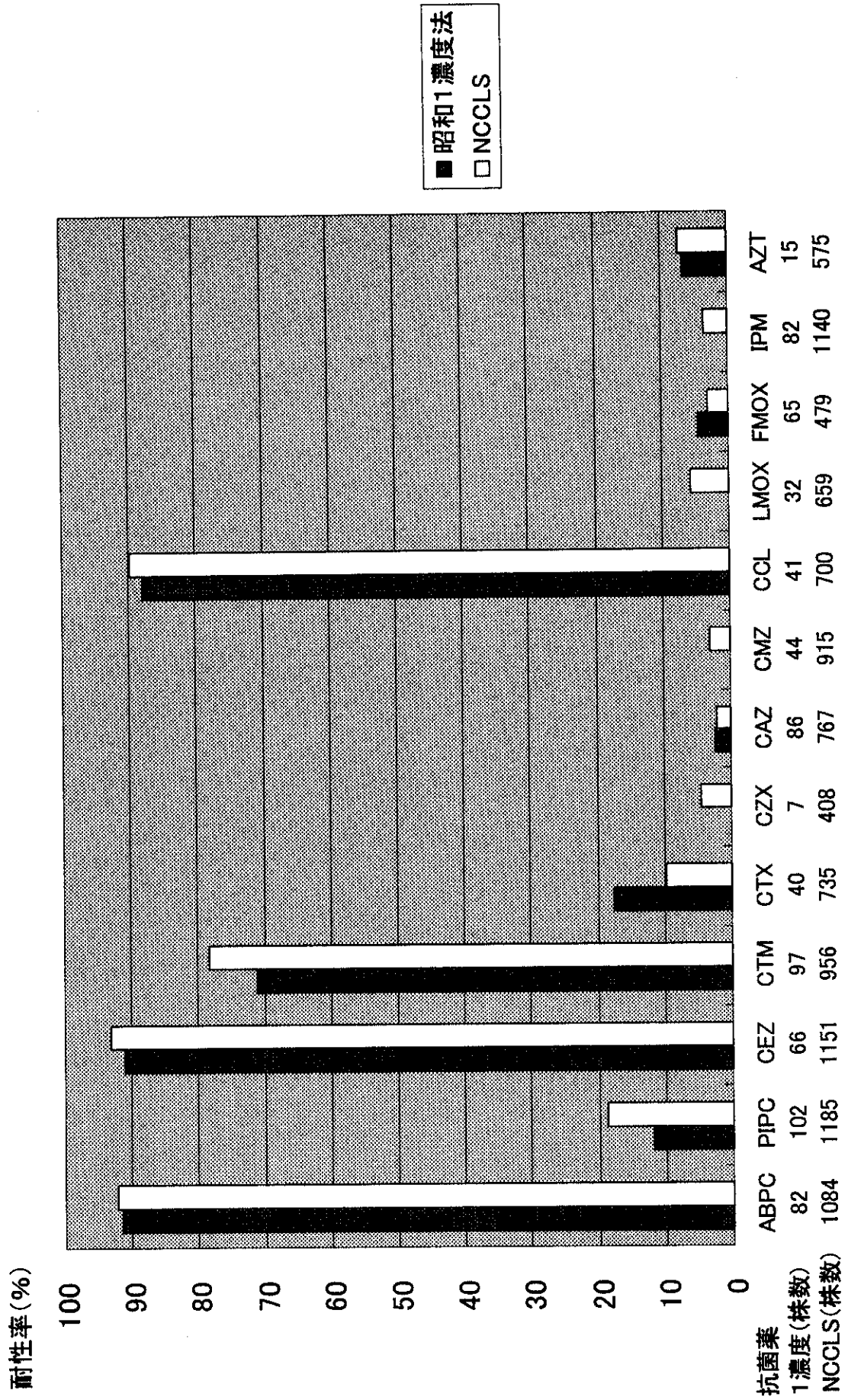
図29—1 Proteus vulgaris
