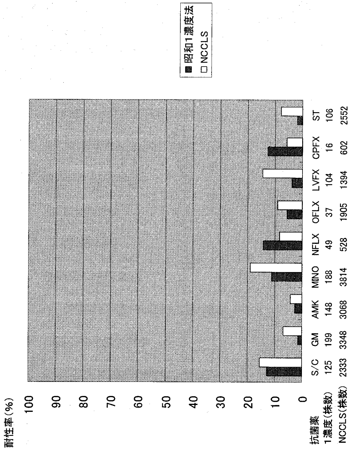
図27-2 Citrobacter freundii
