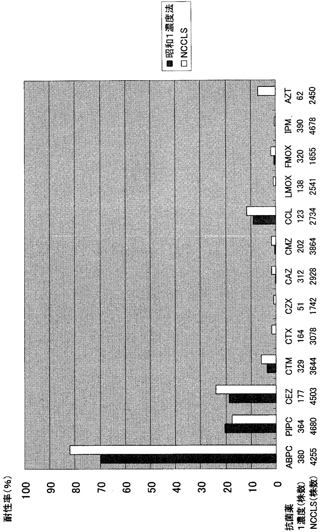
図22-1 Klebsiella oxytoca
