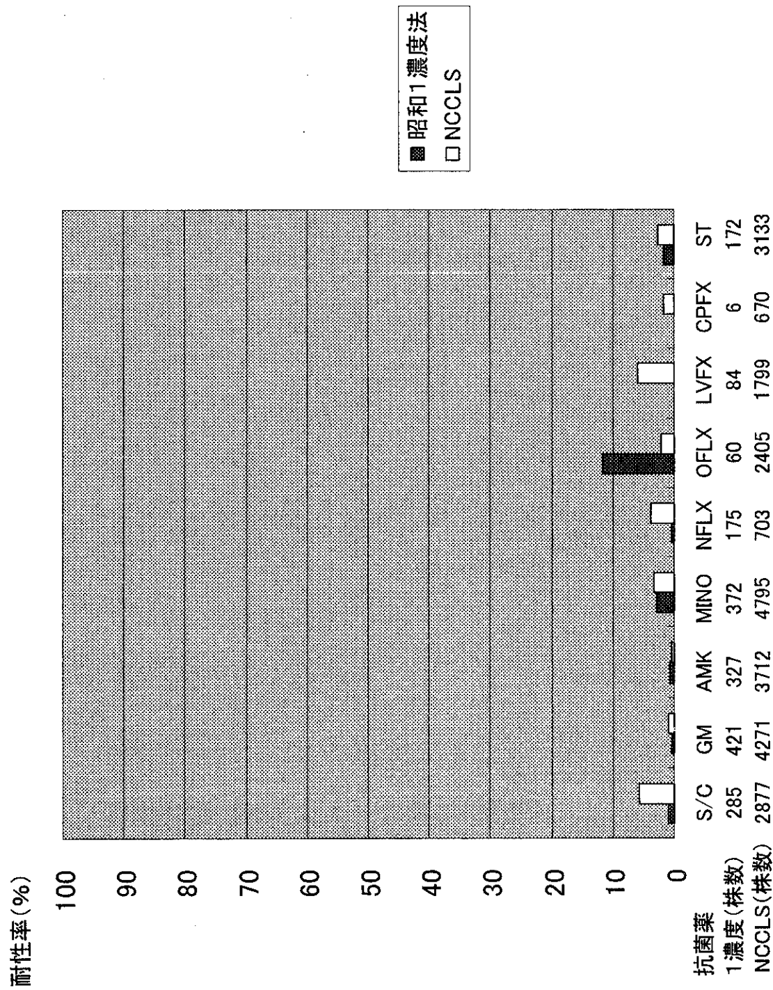
図22-2 Klebsiella oxytoca
