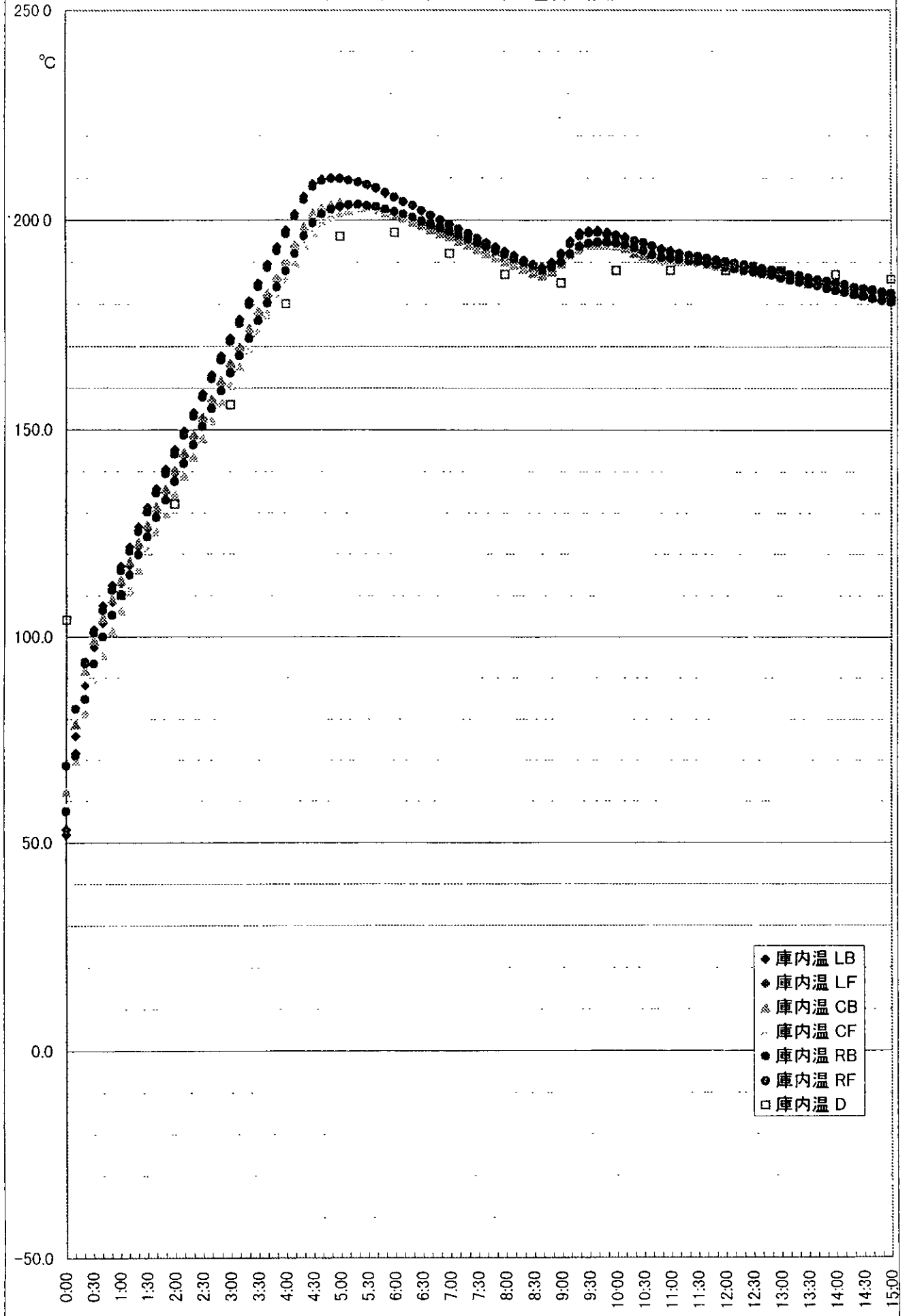
185°C10分加熱後5分放置での庫内温度の推移 1
