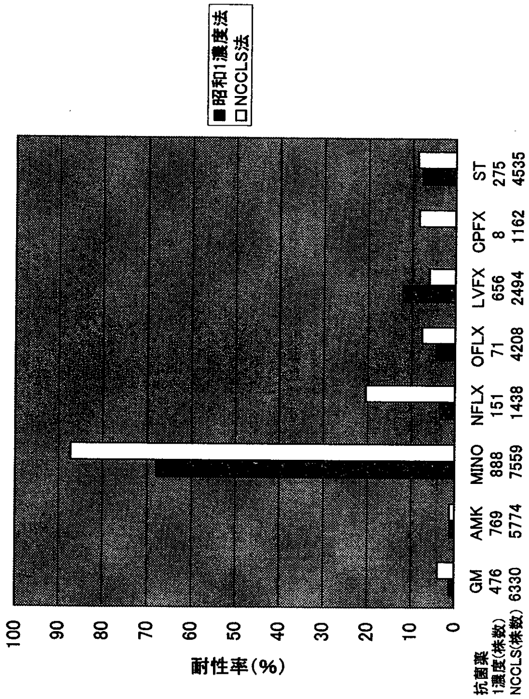
图28-2 Proteus mirabilis
