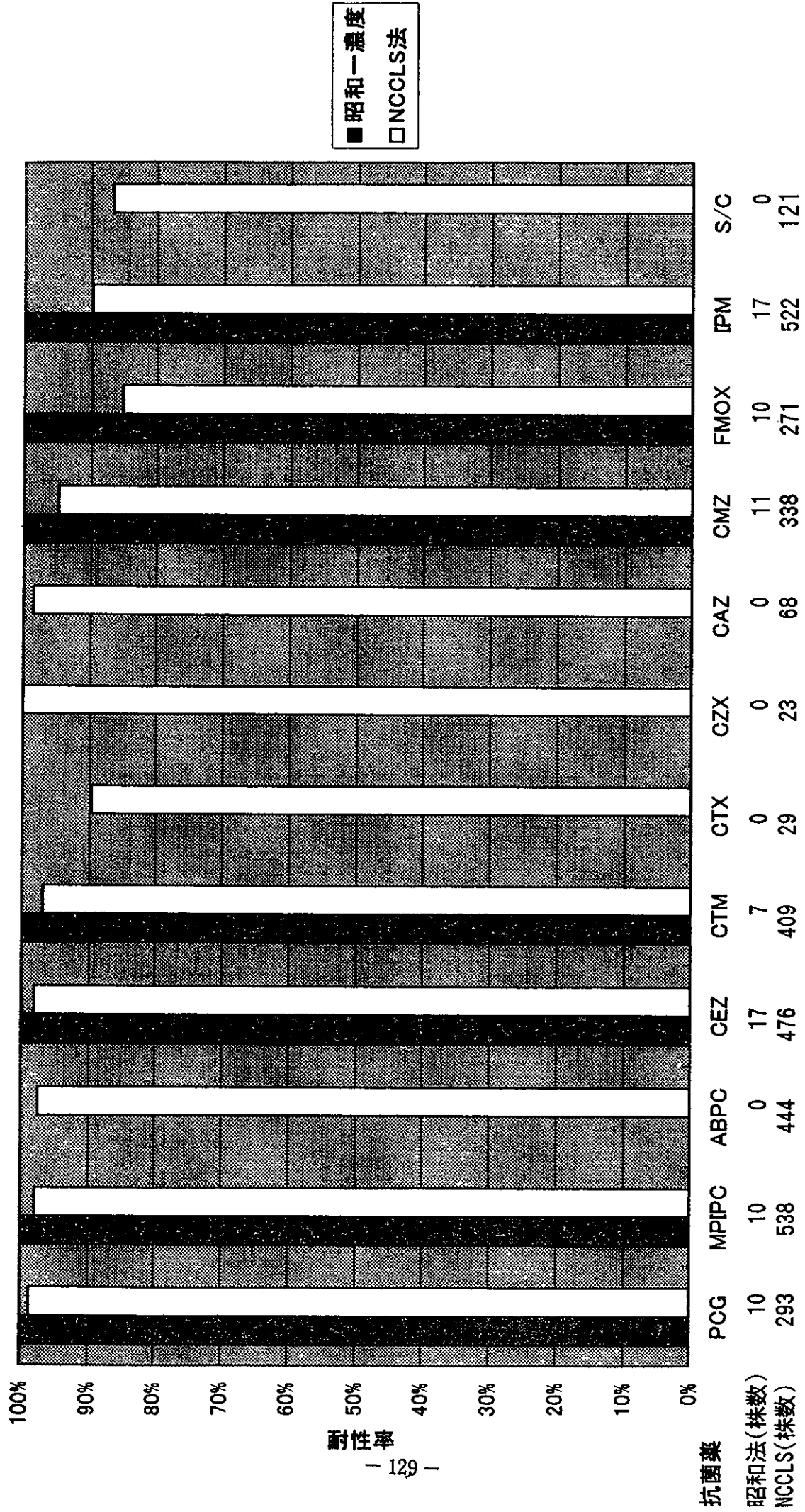
图32-1 MRSA-喹啉
