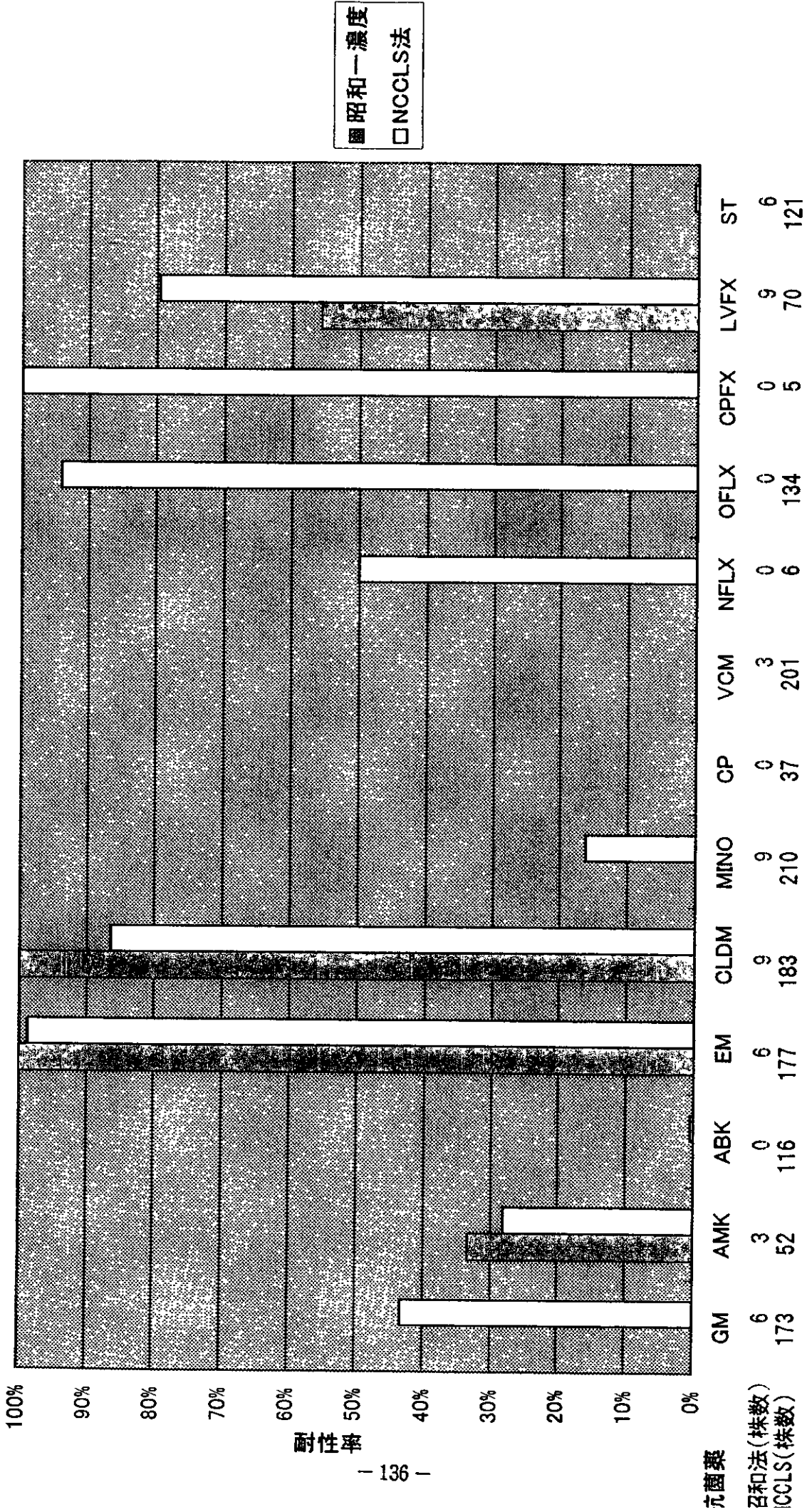
图35-2 MRSA-膜
