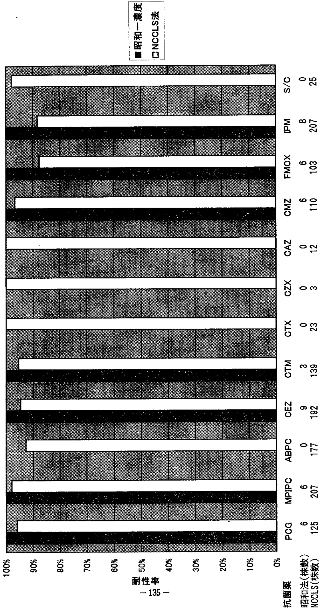
图35-1 MRSA-膿
