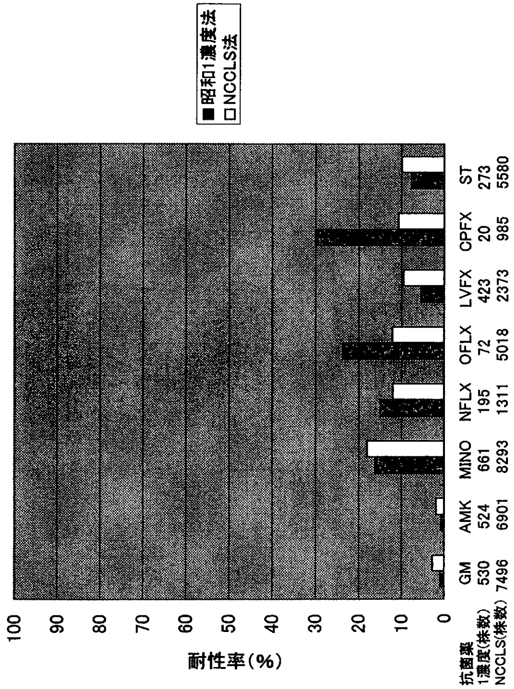
図27-2 Citrobacter freundii
