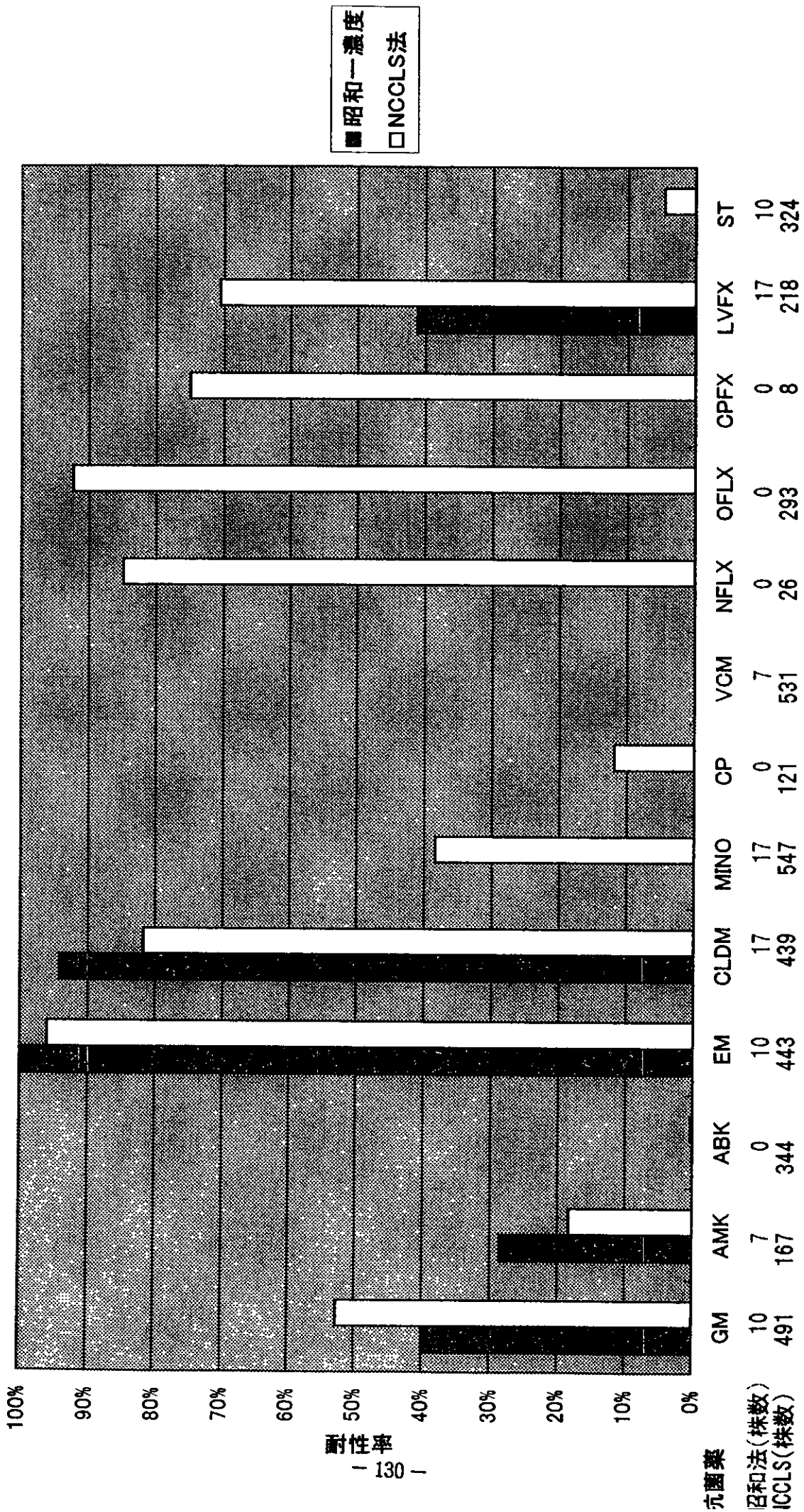
图32-2 MRSA—咯痰
