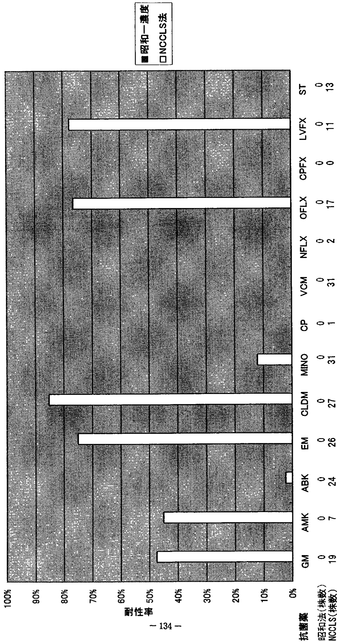
图34-2 MRSA-血液
