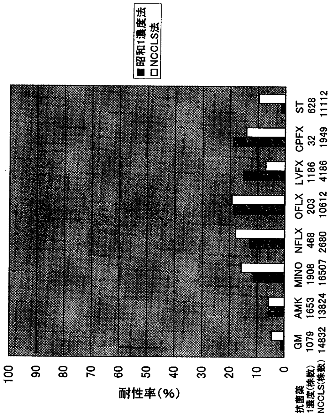
図25-2 Serratia marcescens
